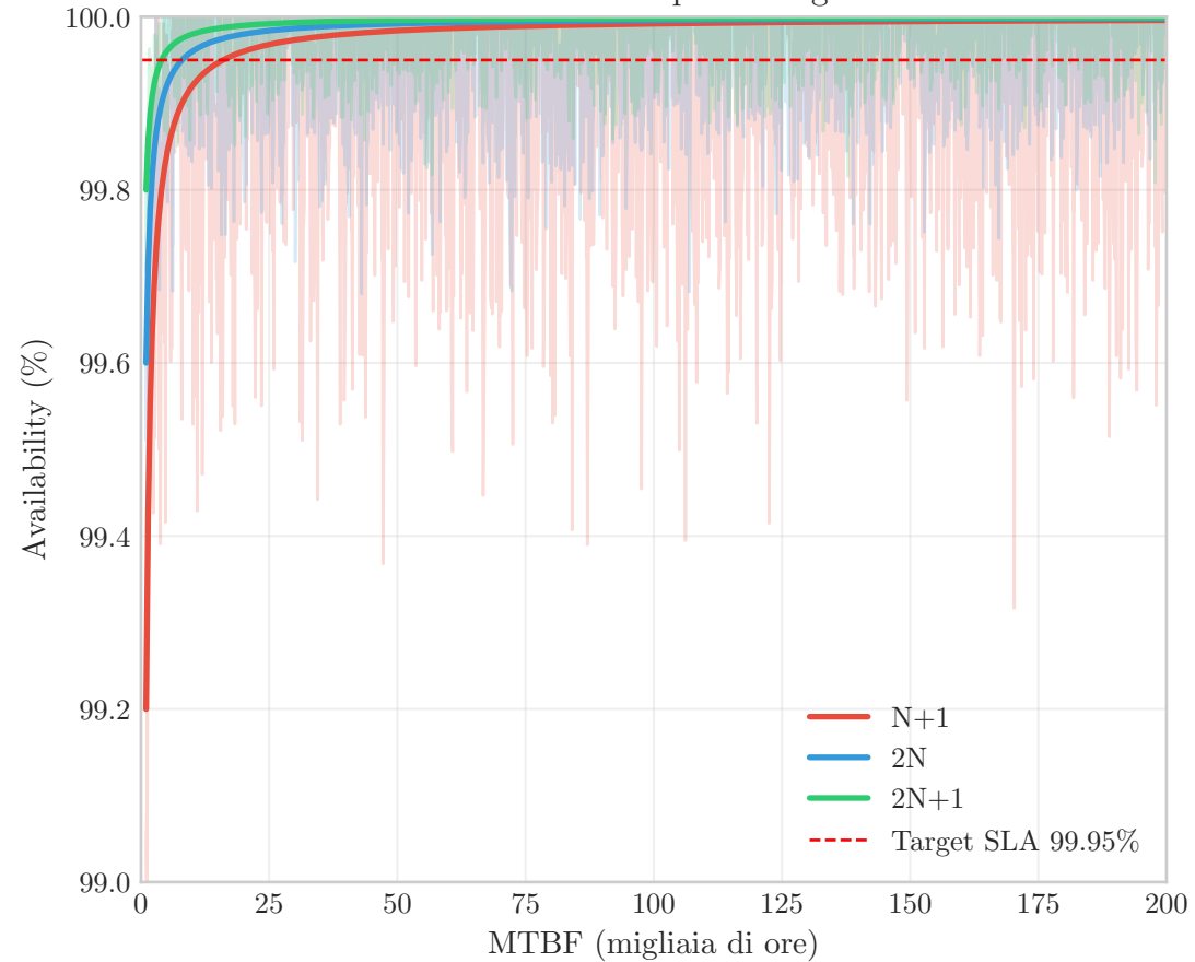
Curve di Affidabilità per Configurazione
