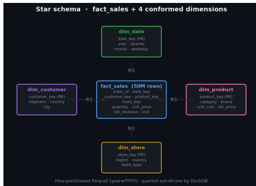
Star schema (data model)
