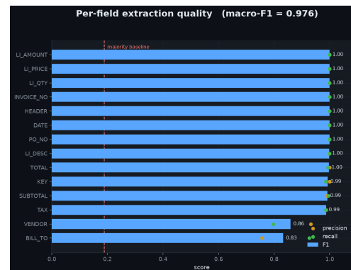
Per-field precision / recall / F1
