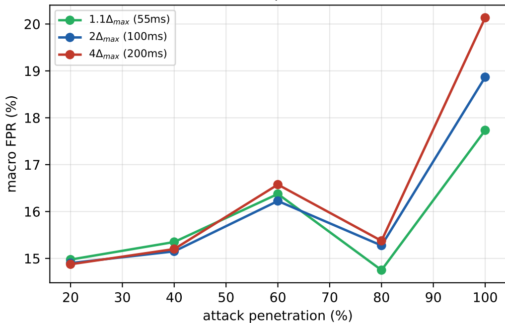
(b) FPR vs penetration
