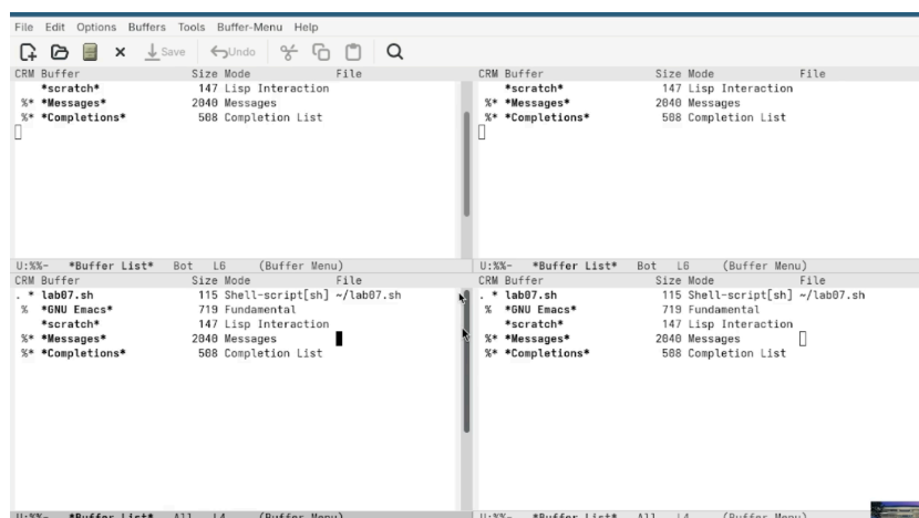
Рис. 5: Фрейм Emacs, разделённый на 4 окна
