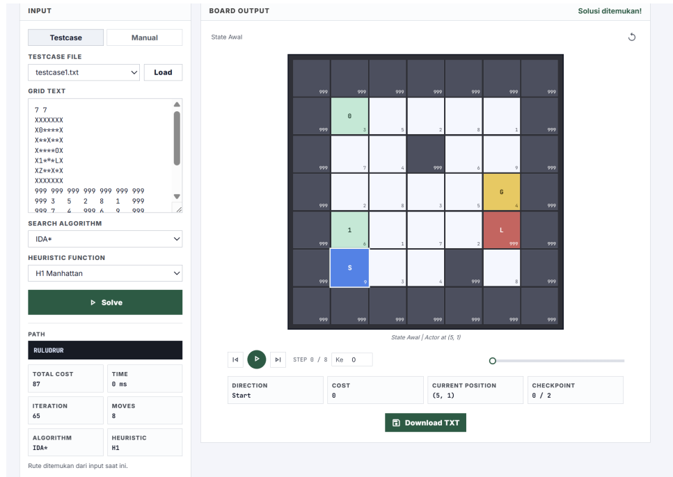
Gambar 4: Testcase 1 dengan IDA*-H1 — total biaya 87, 8 langkah, 65 iterasi. Redundansi komputasi DFS berulang terlihat jelas dibanding A*.
