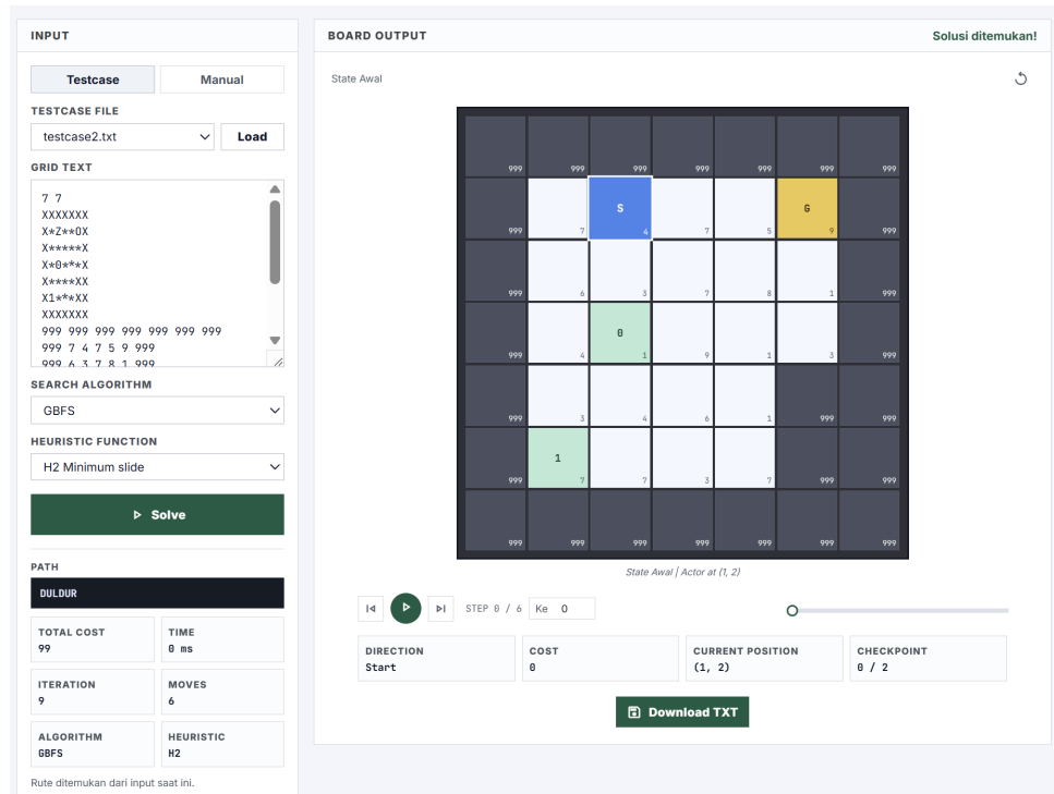
Gambar 6: Testcase 2 dengan GBFS-H2 — total biaya 99, 6 langkah, 9 iterasi. Heuristik H2 menghasilkan rute lebih mahal; GBFS tidak menjamin optimal.
