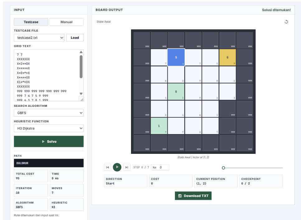
Gambar 7: Testcase 2 dengan GBFS-H3 — total biaya 95, 7 langkah, 10 iterasi. H3 menghasilkan estimasi lebih akurat dari H2 sehingga biaya sedikit lebih rendah.
