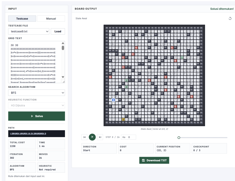
Gambar 12: Testcase 9 dengan BFS — total biaya 1158, 26 langkah, 302 iterasi. BFS menemukan rute dengan jumlah langkah paling sedikit, tetapi biayanya tidak optimal.
