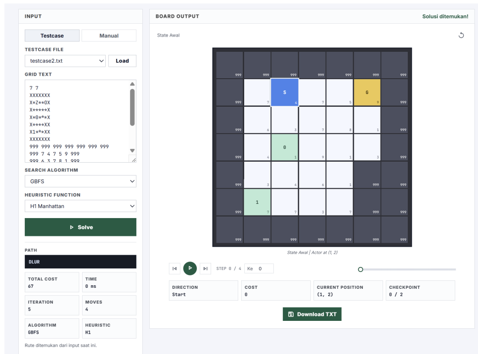
Gambar 5: Testcase 2 dengan GBFS-H1 — total biaya 67, 4 langkah, 5 iterasi. GBFS menemukan rute dengan langkah paling sedikit secara kebetulan pada puzzle kecil ini.
