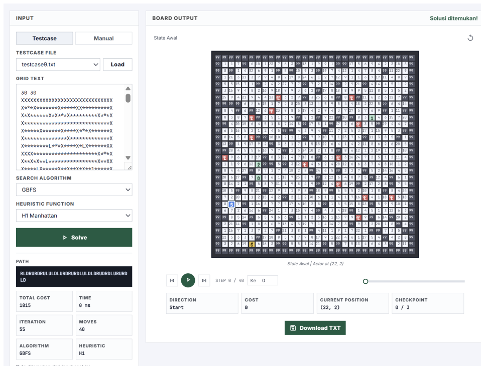
Gambar 13: Testcase 9 dengan GBFS-H1 — total biaya 1815, 40 langkah, 55 iterasi. Ekspansi paling sedikit, namun menghasilkan rute yang jauh dari optimal (+57,9% dari biaya minimum).
