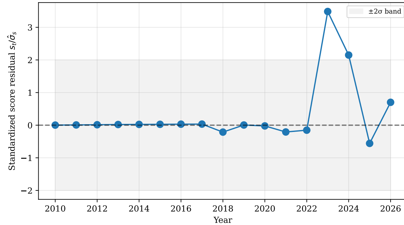
Panel D: AR(1) scatter GAS fit kwaliteit
