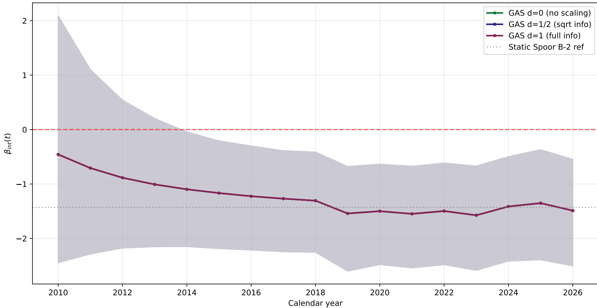
GAS robustness: trajectory voor d \in \{0, 1/2, 1\}
