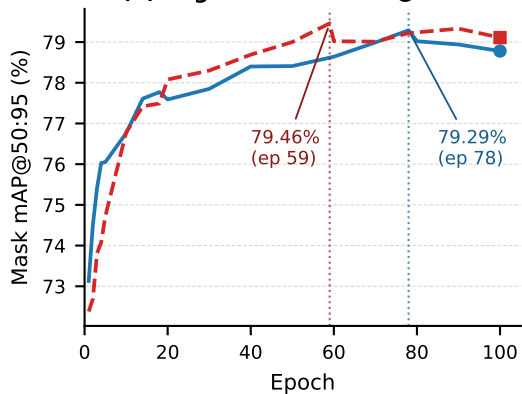
(d) Segmentation mAP@50:95
