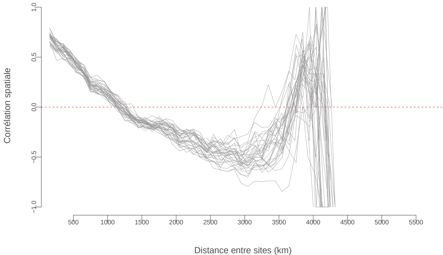
Corrélogramme spatial (autocorrélation des données de présence/absence)
