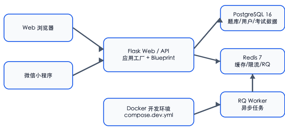
图 1 系统整体架构图
