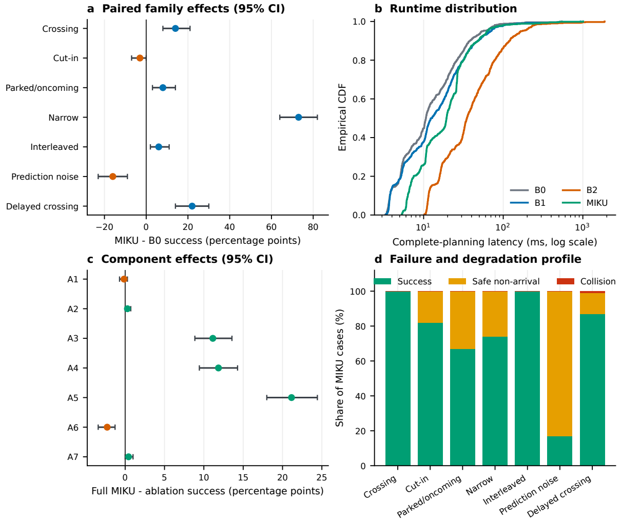
图 2: 由原始 CSV 生成的配对证据总览: (a) MIKU-B0 分场景到达率差及 95% CI; (b) 完整规划耗时 ECDF; (c) 完整 MIKU 相对各消融项的到达率差; (d) MIKU 分场景成功、安全未到达与碰撞构成。
