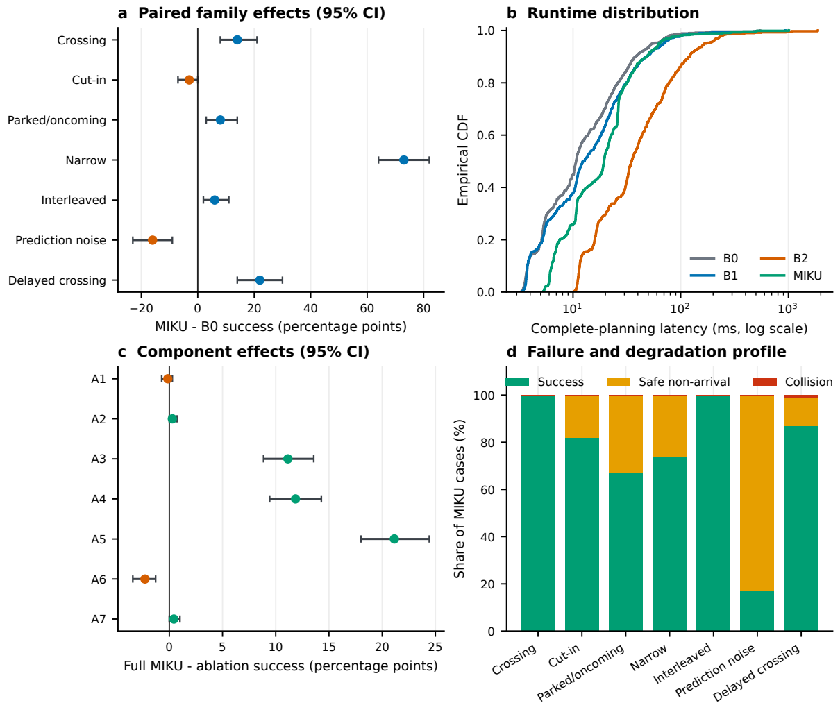
图 3: 由原始 CSV 生成的配对证据总览: (a) MIKU-B0 分场景到达率差及 95% CI; (b) 完整规划耗时 ECDF; (c) 完整 MIKU 相对各消融项的到达率差; (d) MIKU 分场景成功、安全未到达与碰撞构成。
