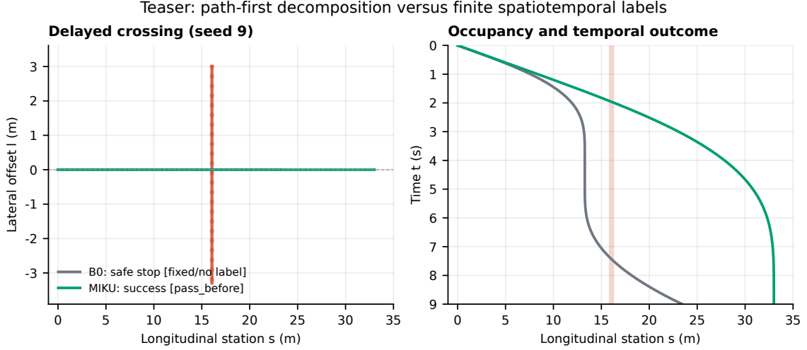
图 1: 首页概念图: 在固定种子的延迟横穿场景中, 时间盲基线 B0 停车, 而 MIKU 保留 pass-before 空间-时间标签并到达目标。左图为 S-L 轨迹, 右图为 S-T 轨迹及障碍物占据。该图由确定性实验重放生成, 用于说明问题机制, 不代表实车部署。
