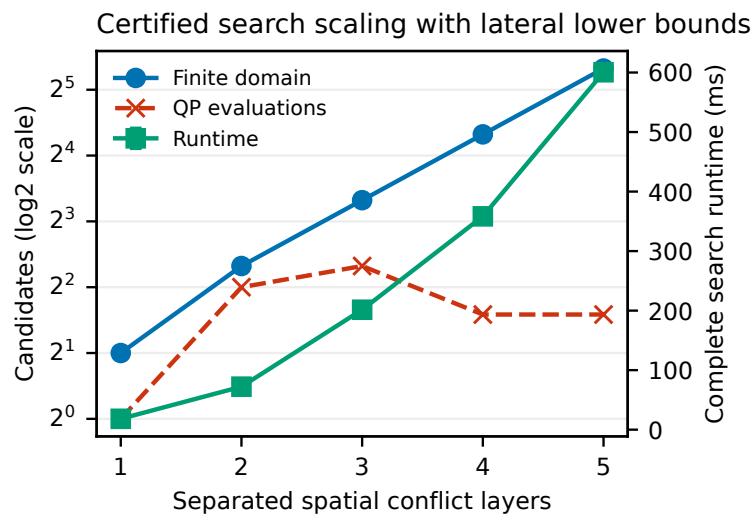
图 5: 非平凡有限联合域的规模诊断。每层含两个可行空间带, 并叠加一个动态横穿。走廊到零线的平方距离提供可采纳下界, 候选域与 QP 评估数的差异直接显示实际剪枝。
