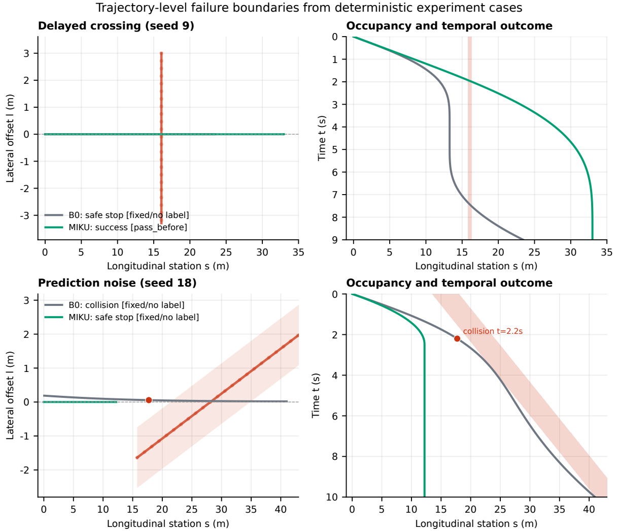
图 4: 由固定种子和同一规划代码生成的轨迹级边界诊断。上行延迟横穿样本中, B0 停车而 MIKU 选择 pass_before 时窗并到达; 下行预测含噪样本中, B0 在 t = 2.2s 碰撞, 而 MIKU 因有限域不可证而安全停车。红色带为真值障碍物占据, 图例同时报告结果、同伦标签和证书状态。该图是算法级仿真诊断, 不是实车或 Apollo/CyberRT 轨迹。
