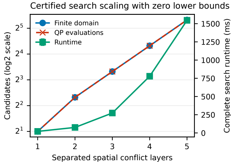
图 4: 非平凡有限联合域的规模诊断。每层含两个可行空间带，并叠加一个动态横穿。候选域与 QP 评估数重合，说明当前零下界不产生剪枝。
