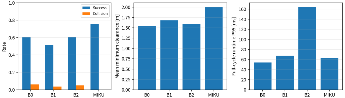
图 2: 7 类配对随机场景的总体性能
