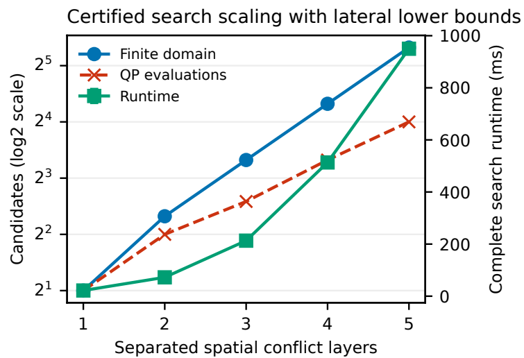
图 5: 非平凡有限联合域的规模诊断。每层含两个可行空间带, 并叠加一个动态横穿。空间分支的路径 QP 最优值提供可采纳下界, 候选域与 QP 评估数的差异直接显示实际剪枝。
