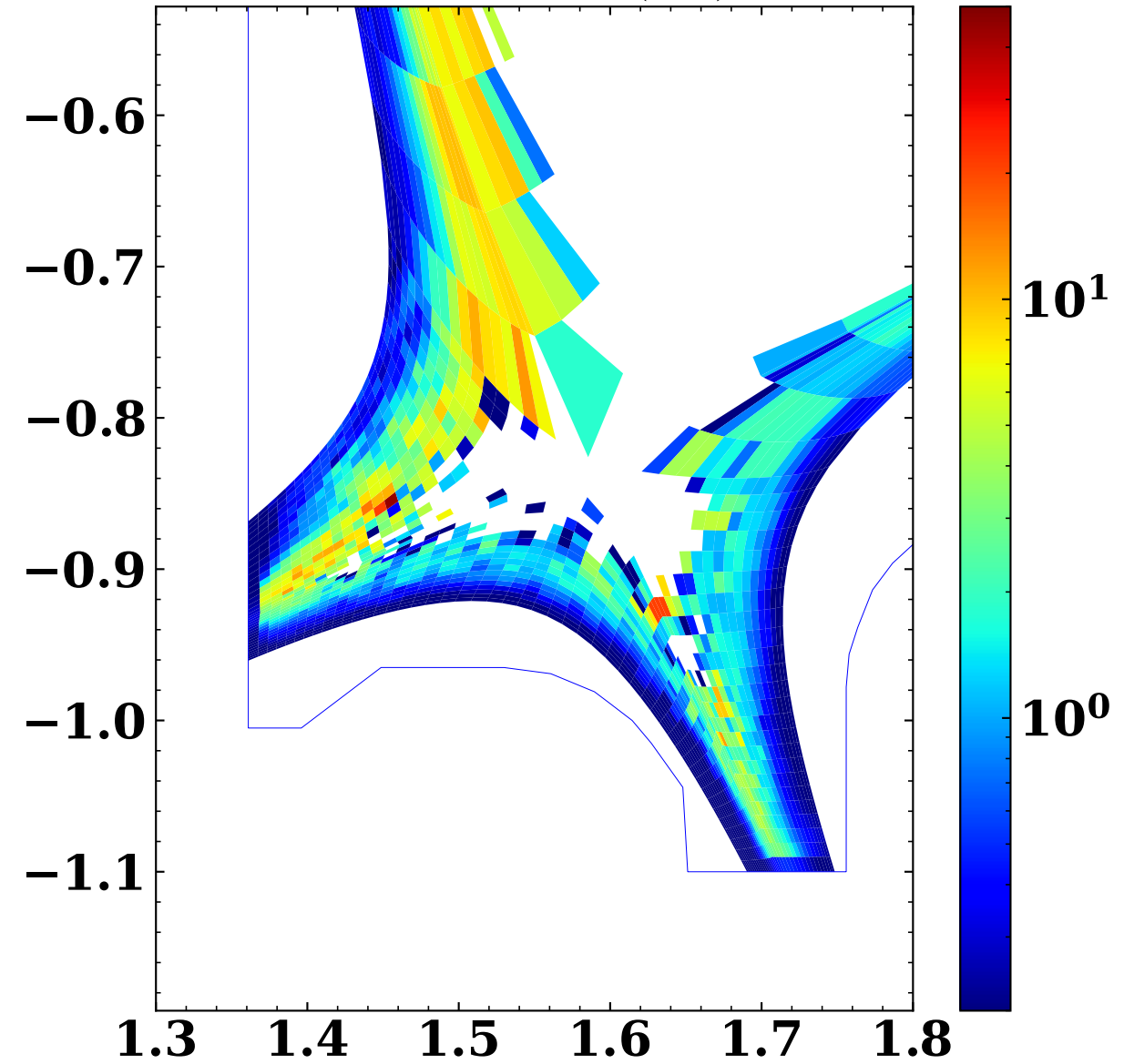
4e19 T_{D2^0} (eV)
