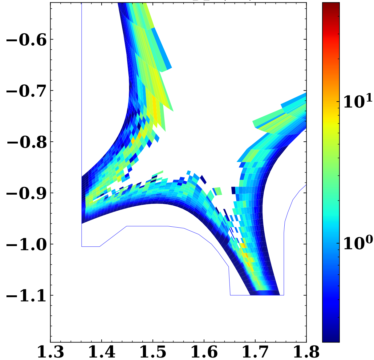
4.6e19 T_{D2^0} (eV)
