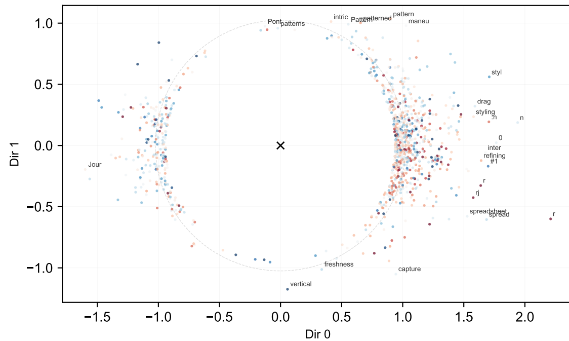
M1 — L58 o_proj s0=3.60
