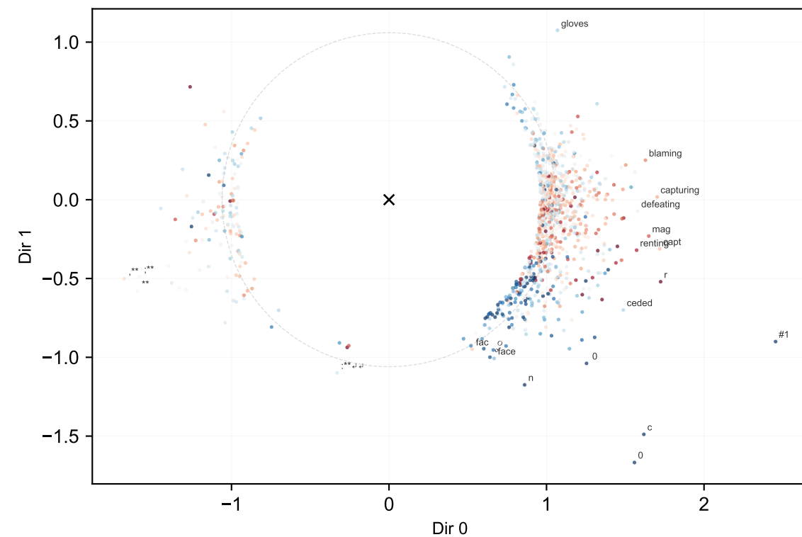
M1 — L60 o_proj s0=3.45
