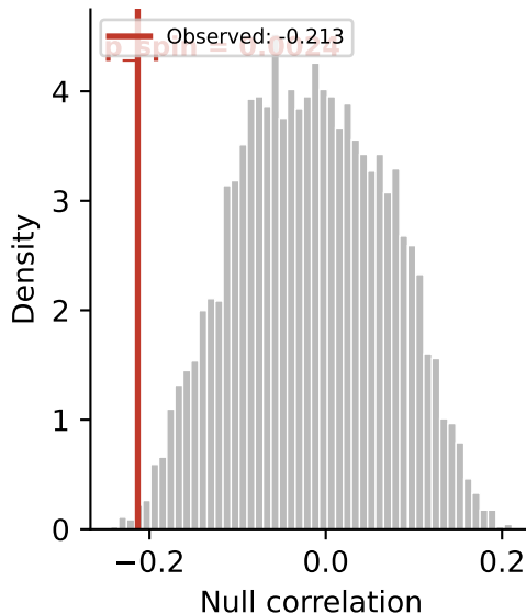
SCov G2 | z
