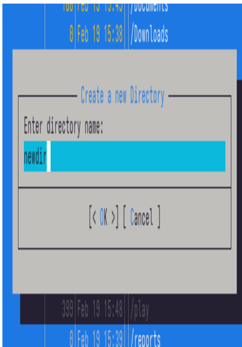
Рисунок 2.12: Создание каталога
