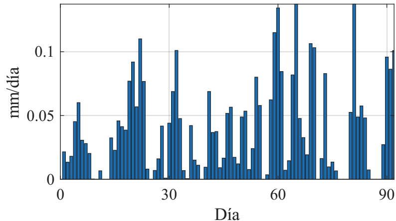
Precipitación diaria
