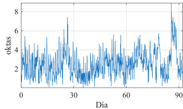
Nubosidad diaria
