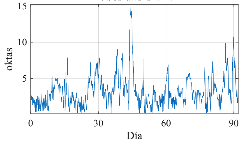
Nubosidad diaria
