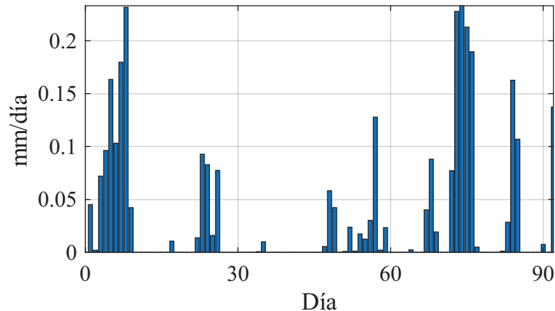
Precipitación diaria
