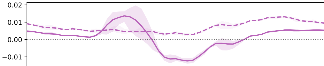
Zooplankton
