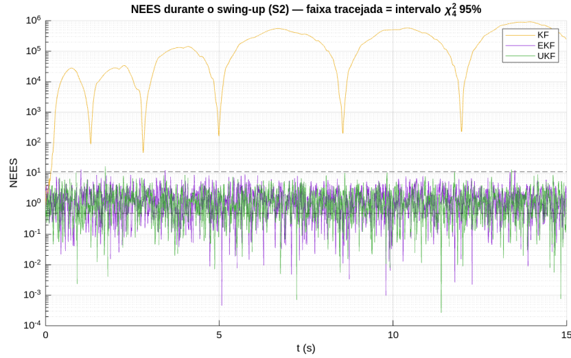
Figura 5: NEES ao longo do swing-up (S2) para KF, EKF e UKF (escala log). A faixa tracejada é o intervalo \chi_4^2 a 95%, [0,48; 11,14] . O KF passa a maior parte do tempo quatro a cinco ordens de grandeza acima do limite superior — o próprio filtro "acredita" ter convergido (sua covariância P encolhe) ao mesmo tempo em que o erro real explode, o padrão clássico de divergência otimista de um filtro linear fora de sua região de validade. EKF e UKF permanecem dentro (ou muito perto) da faixa esperada o tempo todo.
