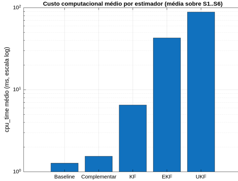
Figura 6: Custo computacional médio por estimador ( cpu_time , escala log), medido dentro de run_scenario.m e médio sobre os seis cenários. A ordem reflete diretamente a complexidade algorítmica de cada método por passo: baseline e complementar são O(1) (sem álgebra matricial); KF é uma predição/atualização 4 \times 4 fixa; EKF soma o custo de jacobian_f + expm ( 4 \times 4 ) a cada passo; UKF paga por 2n+1 = 9 integrações RK4 completas da dinâmica não-linear por passo, além da fatoração de Cholesky.
