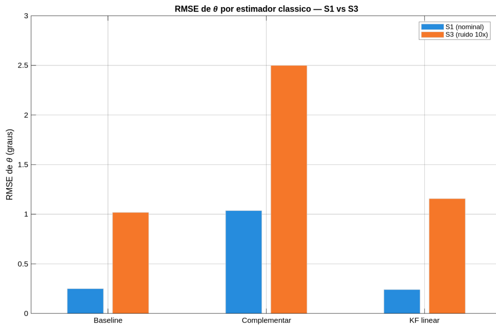
Figura 3: RMSE de \theta dos três estimadores clássicos no cenário de demonstração, com ruído nominal e com ruído 10\times (análogo a S1 vs. S3). O complementar tem a maior degradação relativa; baseline e KF permanecem próximos em ambos os níveis.
