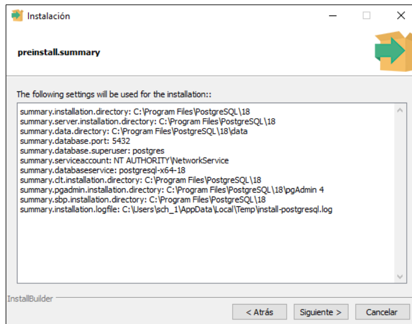
Figura8. Resumen previo a la instalación.
