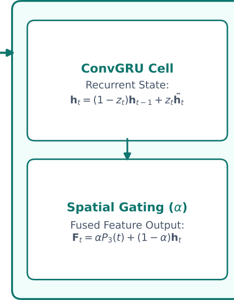
(d) ConvGRU Aggregator
