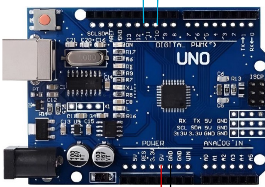
Arduino Uno
