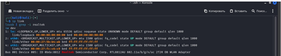
Рис. 1. Адаптер опознан системой: lsusb показывает 0bda:8812 Realtek RTL8812AU
