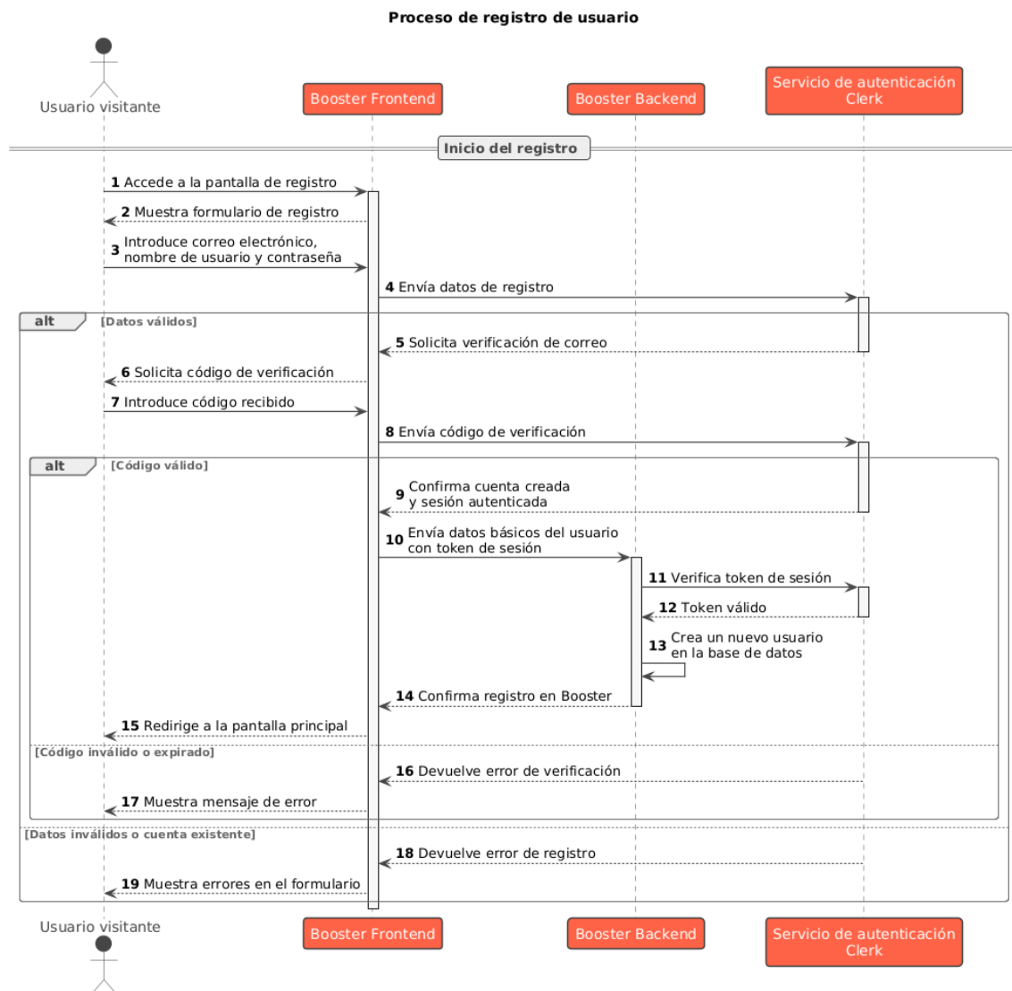
Figura 5.10: Registro - Diagrama de Secuencia
