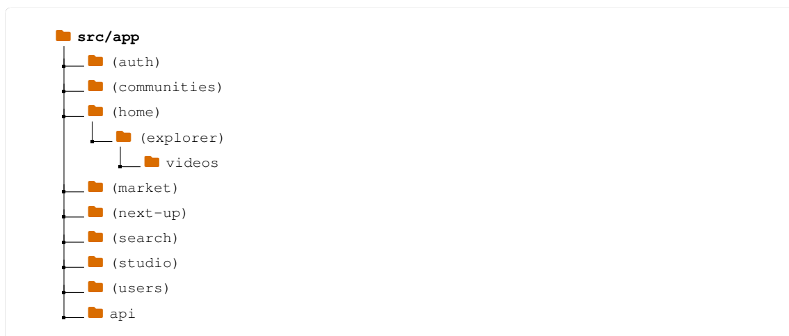
Figura 6.2: Estructura de rutas de la aplicación - Directorio /src/app
