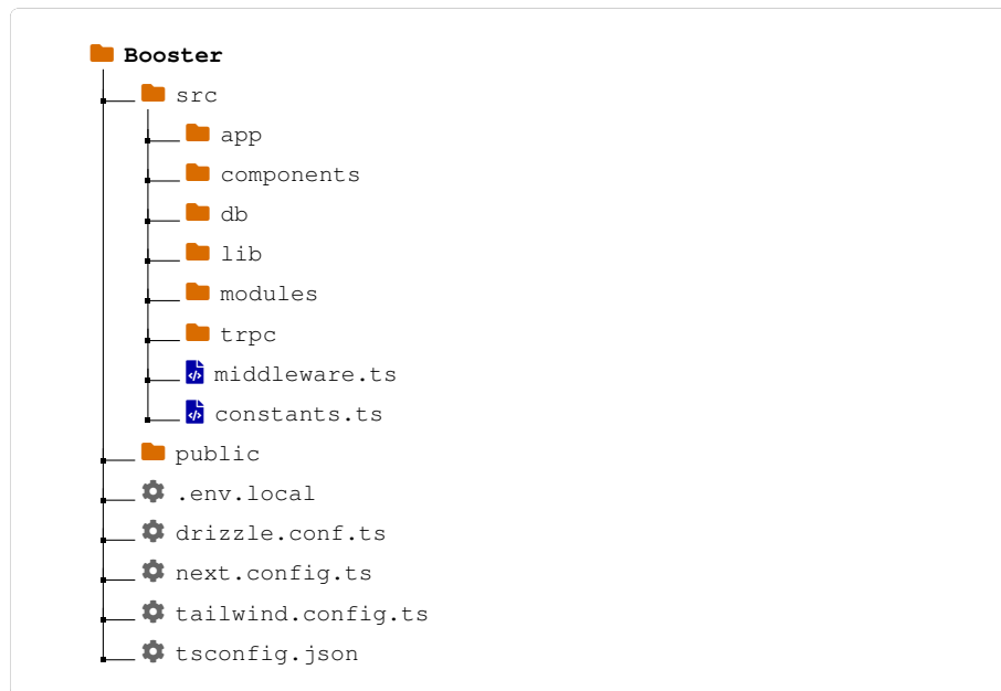
Figura 6.1: Estructura general del proyecto Booster
