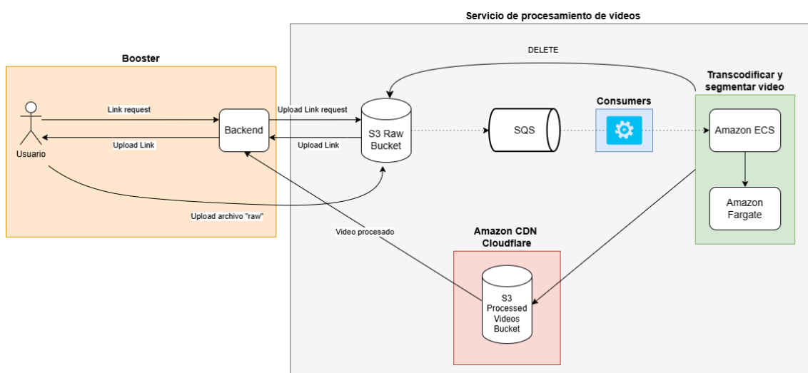
Figura 6.5: Arquitectura de Procesamiento con servicios de Amazon Web Services
