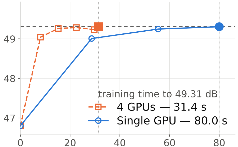
SPERR + Ours — Miranda
