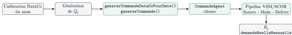
Figure 6 – Injection de la demande DataCo dans le pipeline validé, jusqu’au signal R_j consommé par le Recalibrator.
