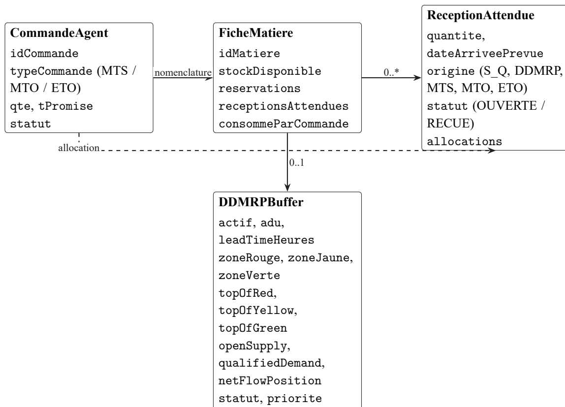
FIGURE 5.1 – Vue simplifiée des classes : la fiche matière possède le stock, les réservations, les réceptions attendues et, optionnellement, le buffer DDMRP.
