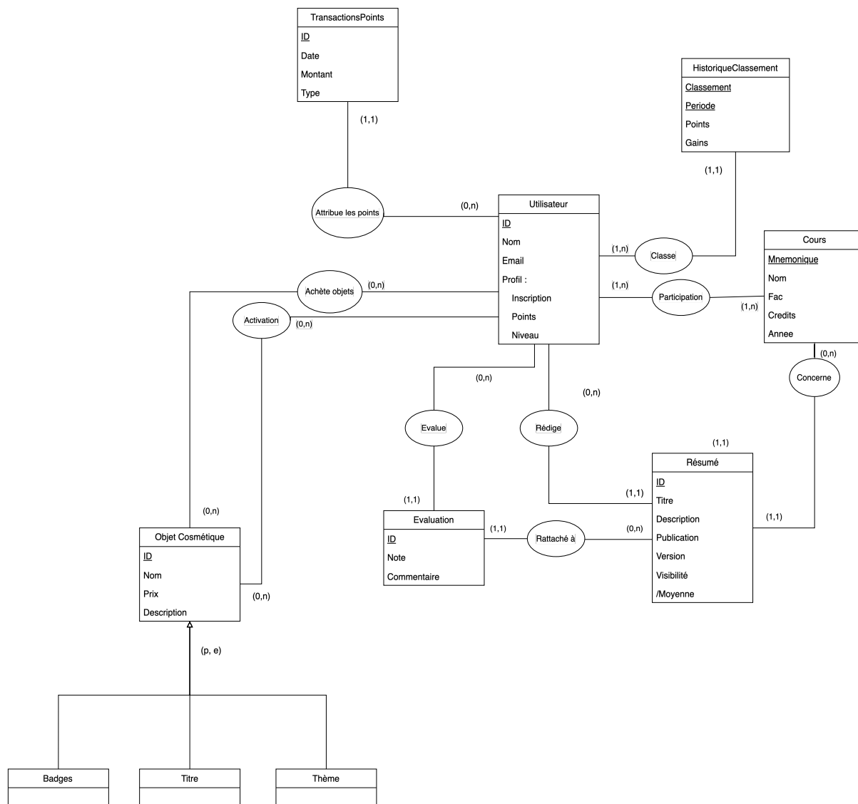
Fig. 2.1. – Diagramme Entité-Association
