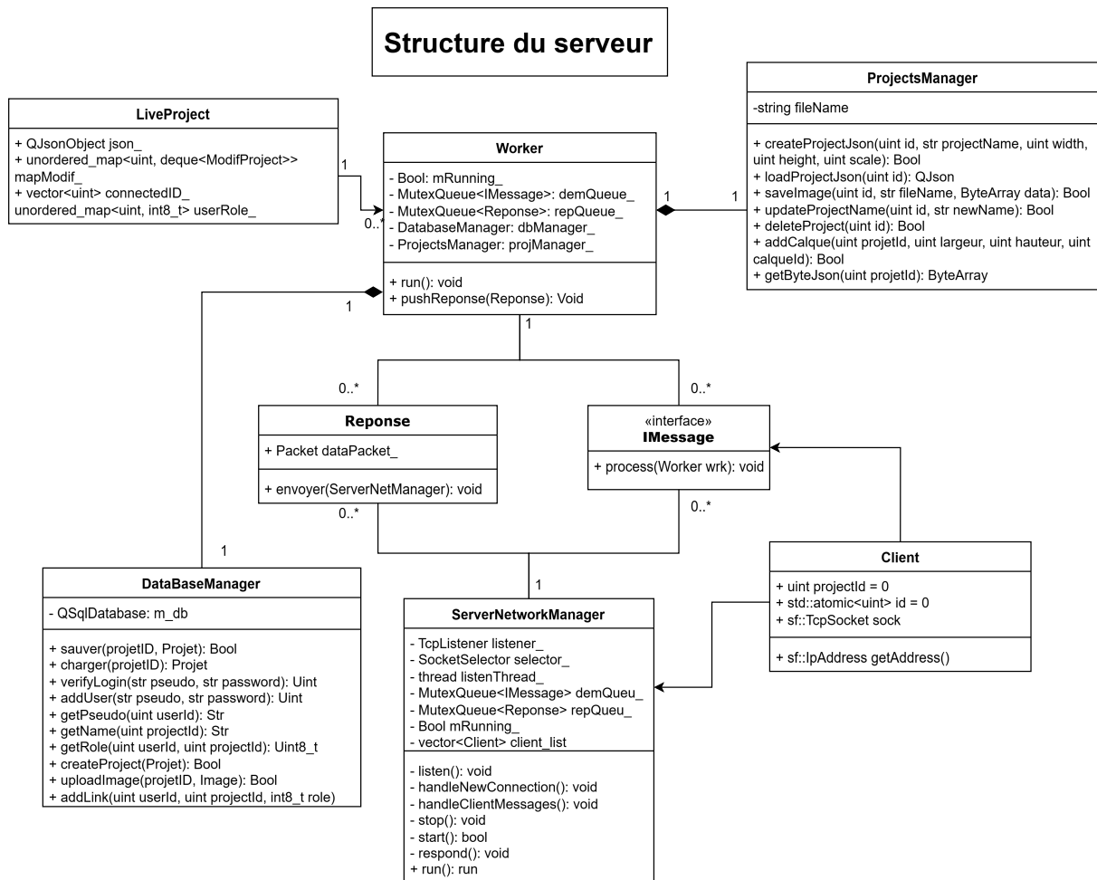
Fig. 2.1. – Diagramme de classe du serveur
