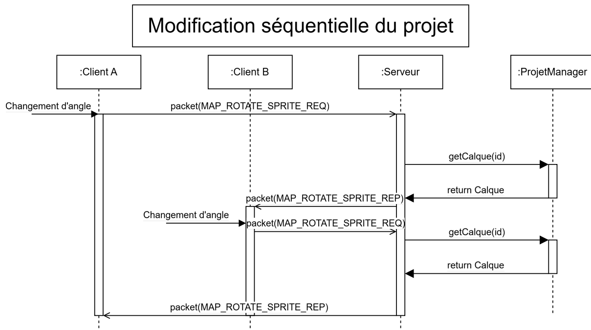
Fig. 5.3. – Diagramme de séquence sur les modification d'un projet
