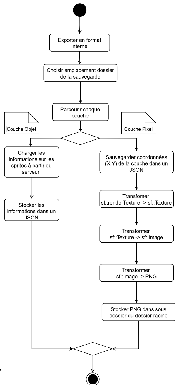
Fig. 3.4. – Exportation d'un projet au format interne
