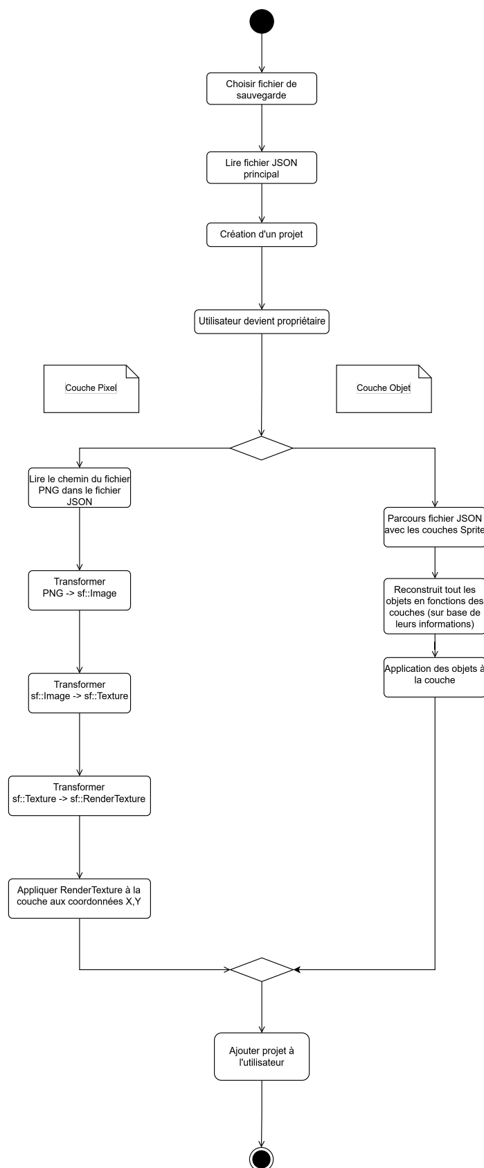
Fig. 3.5. – Importation d'un projet au format interne
