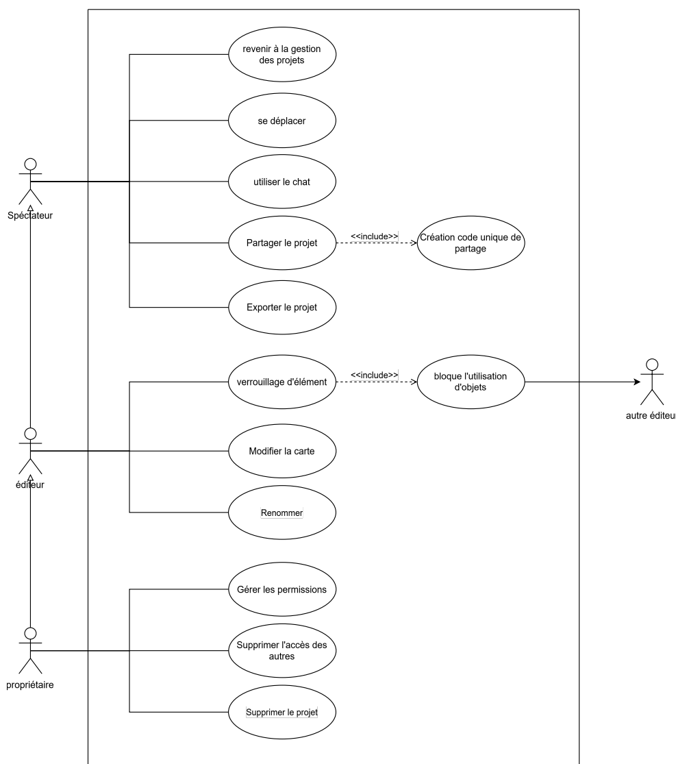
Fig. 3.7. – Use case illustrant les actions possible dans un projet
