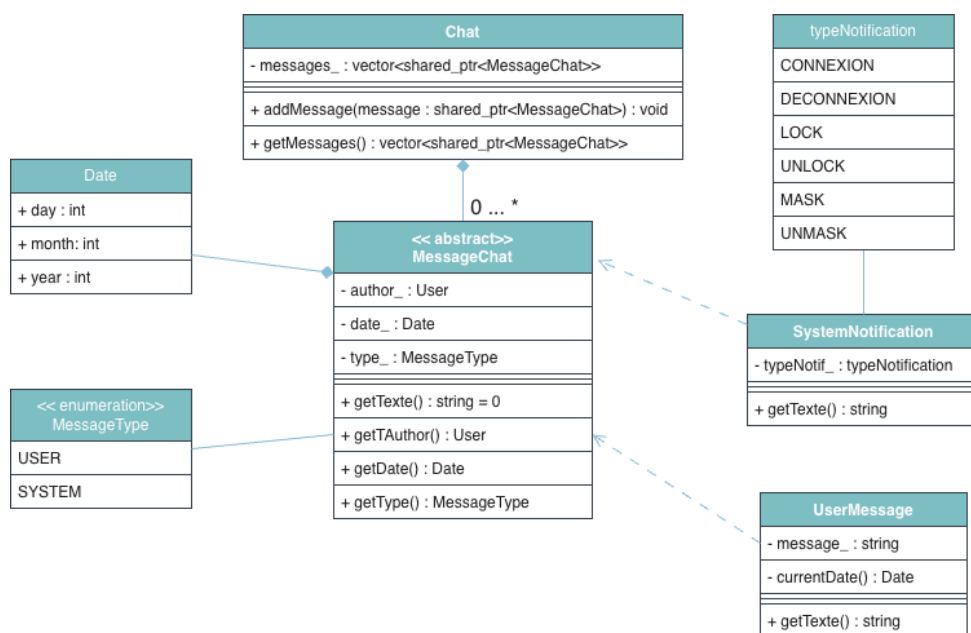
Fig. 3.8. – Diagramme de class pour les messages
