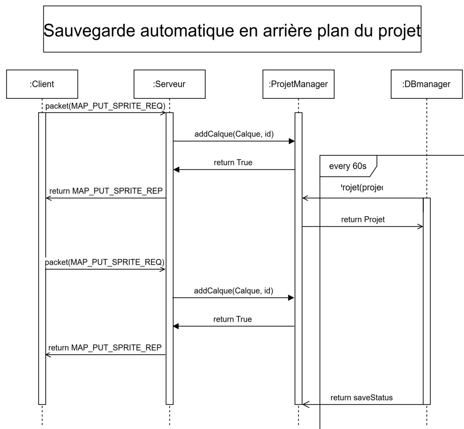
Fig. 5.1. – Diagramme de séquence de la sauvegarde automatique
