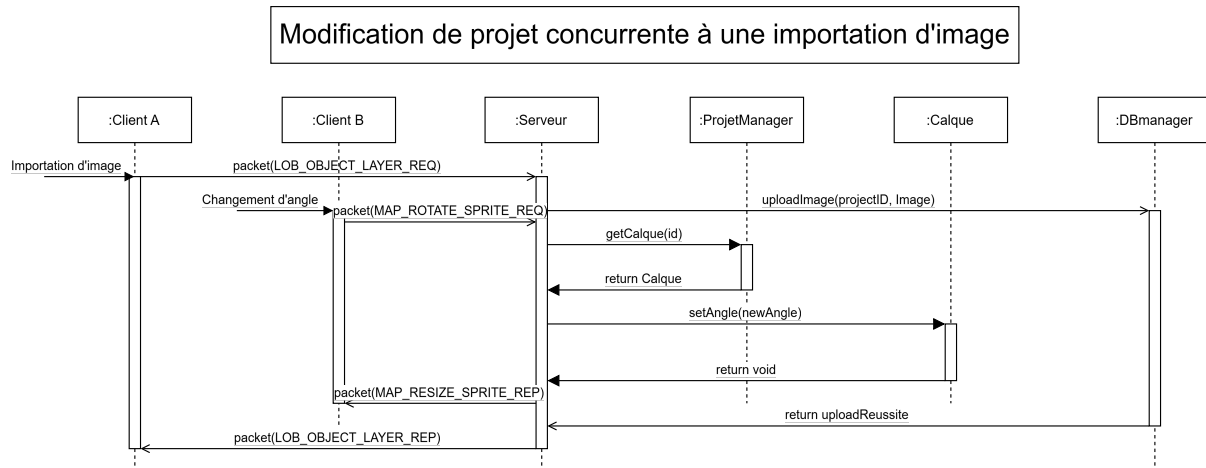
Fig. 5.2. – Diagramme de séquence de l'importation d'image
