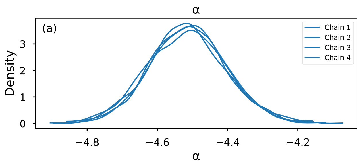
Posterior distributions
