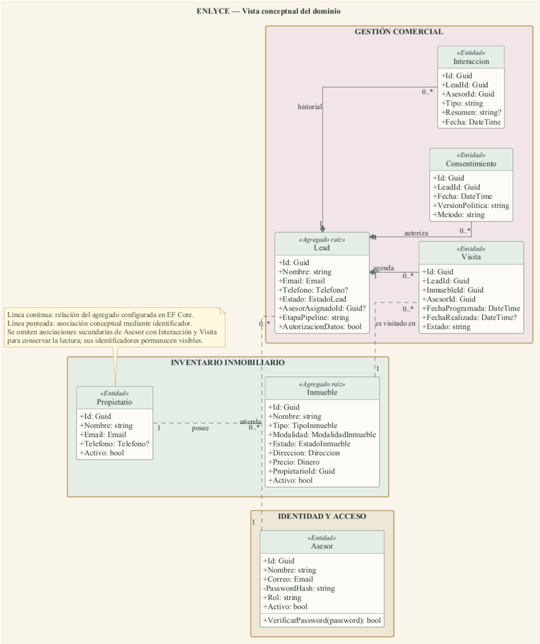
Figura 3. Vista conceptual del dominio organizada por agregados.
