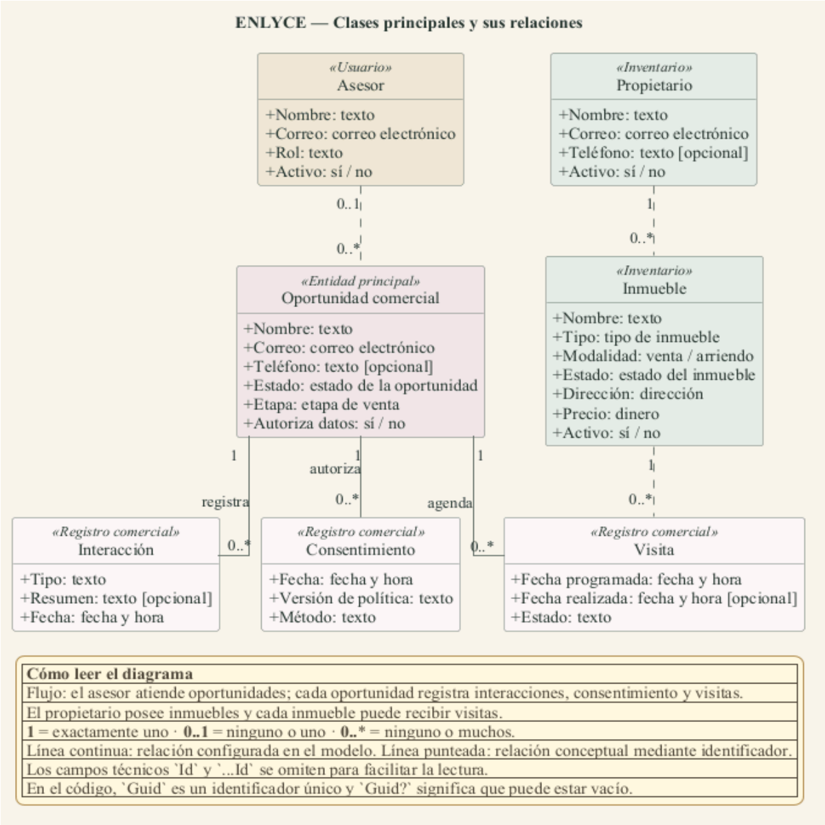
Figura 3. Clases principales de ENLYCE organizadas como flujo de negocio.
