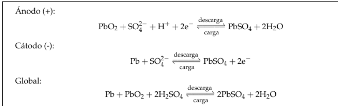
Figura 3.12 Formula química del proceso de descarga y carga de una batería de ácido-plomo
