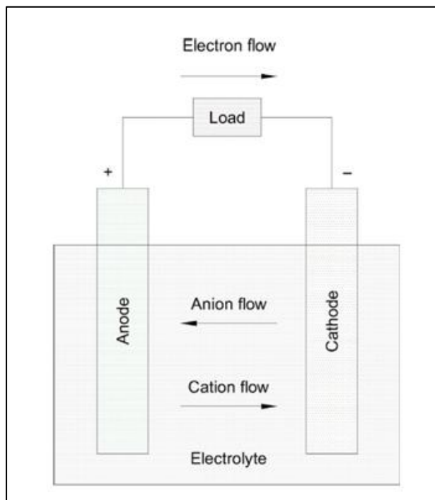
Figura 3.11 Principio de Operatividad de una batería
