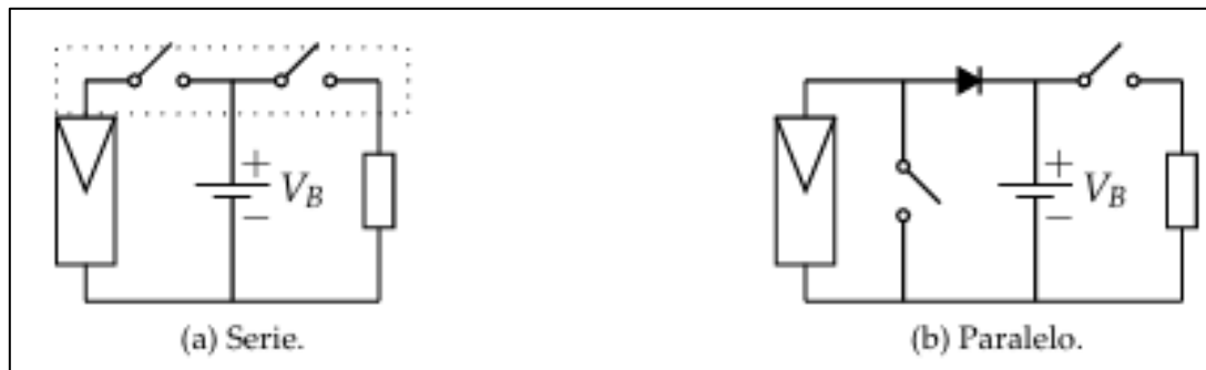
Figura 3.5 Esquema eléctrico de un regulador de carga
