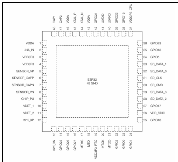
Figura 4.6 Distribución de pines del ESP32
