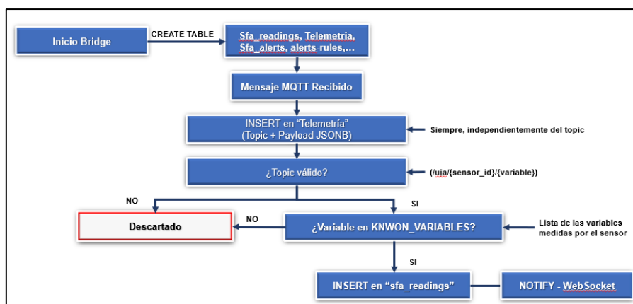
Figura 6.3 Diagrama de procesamiento de datos en el Bridge
