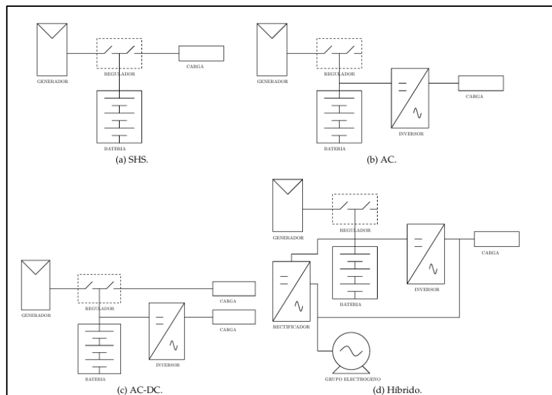
Figura 3.1 Configuraciones típicas de una SFA
