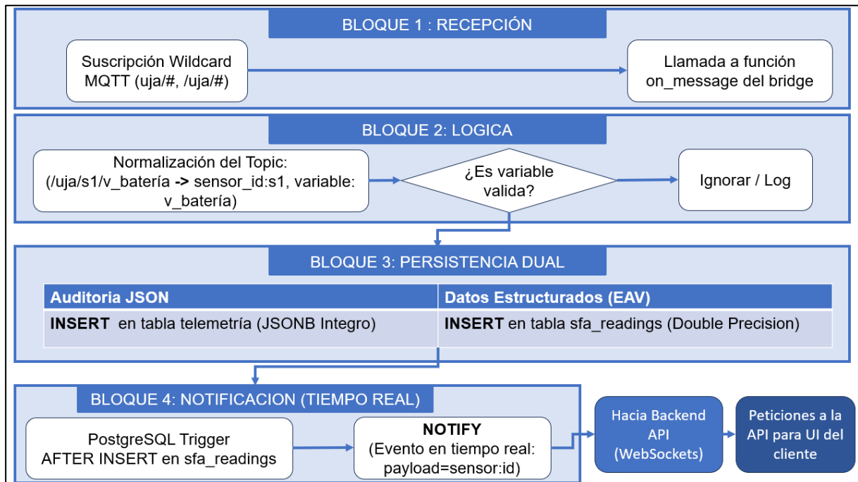
Figura 6.1 Diagrama de procesamiento de datos en el Bridge MQTT (Híbrido Event-Driven)
