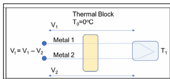
Figura 4.7 Esquemático de una Termocupla
