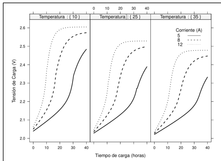
Figura 3.16 Curvas de evolución de la tensión en bornes de una batería durante un proceso de carga a corriente constante, para diferentes valores de corriente de carga y temperatura ambiente (batería de capacidad C10)
