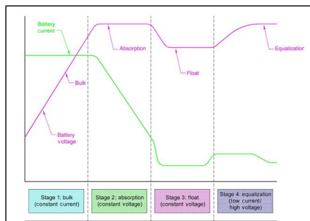
Figura 3.10 Etapas de carga de una batería de plomo-ácido.
