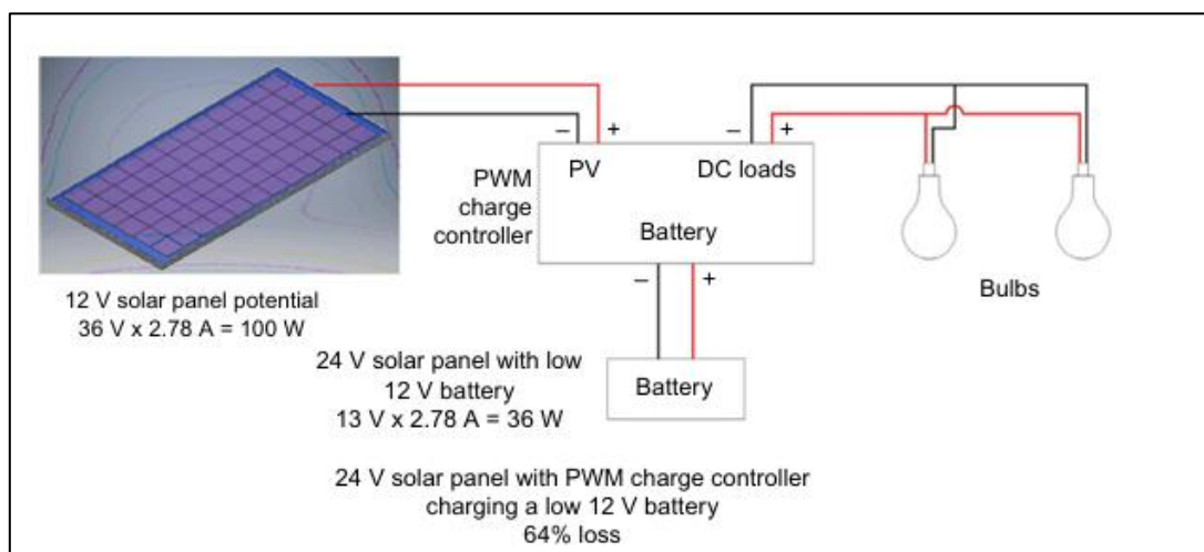
Figura 3.8 Pérdida de energía en una conexión de un módulo de 24V con una batería de 12V con un regulador de carga PWM
