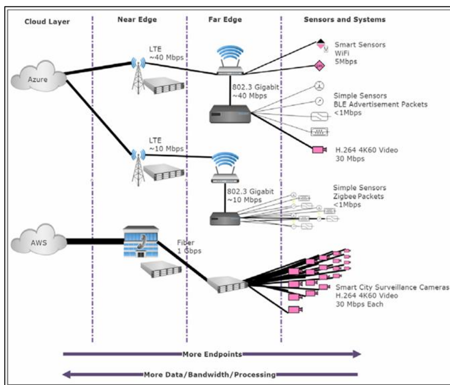
Figura 4.2 Diferencia de proximidad y recursos entre cómputo cercano al borde (Near-Edge) y lejano al borde (Far-Edge)
