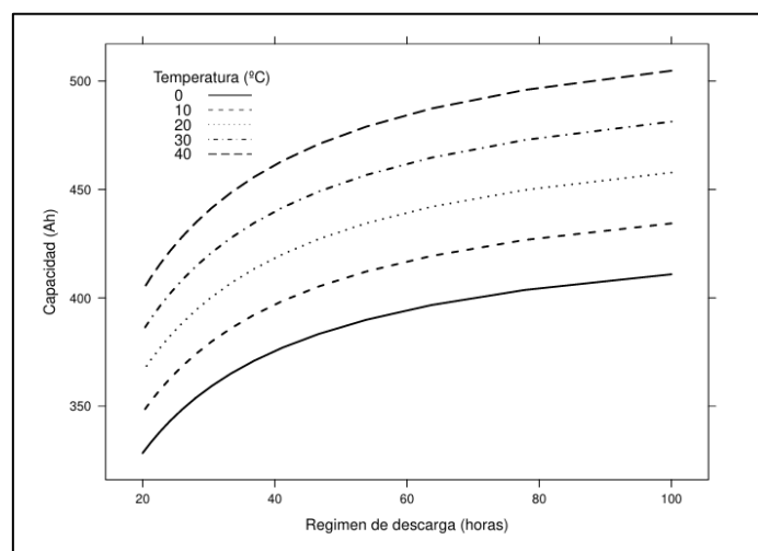
Figura 3.15 Relación entre el régimen de descarga y la capacidad de la batería.
