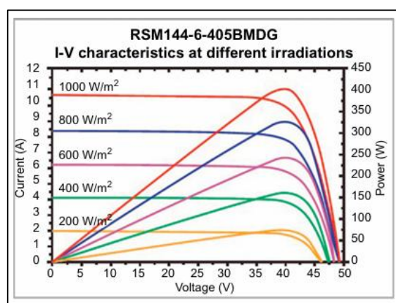
Figura 3.3 Curvas de Corriente-Voltaje y Potencia-Voltaje para diferentes condiciones de irradiancia solar de un módulo de 405W
