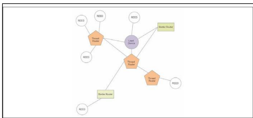
Figura 4.13: Topología de Red Thread
