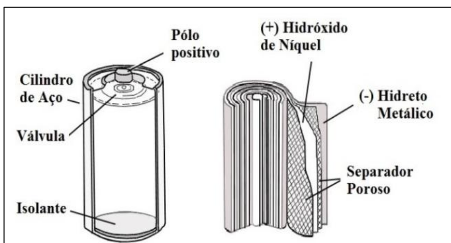
Figura 3.18 Batería cilíndrica de NiMh
