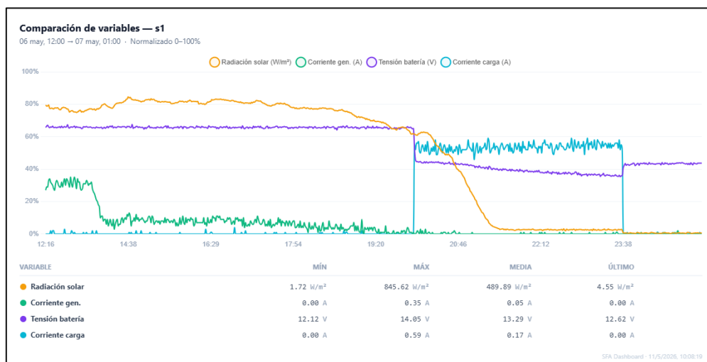
Figura 6.58 Evolución de la tensión durante la descarga
