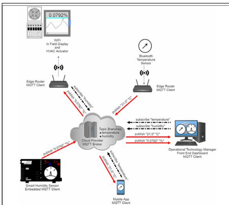
Figura 4.15: Topología y modelo de publicación y suscripción de MQTT
