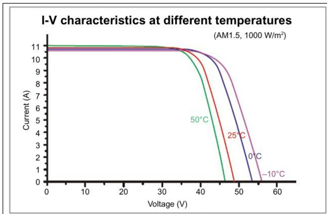
Figura 3.4 Curvas de Corriente-voltaje para un módulo de 405 \text{ W} a diferentes temperaturas
