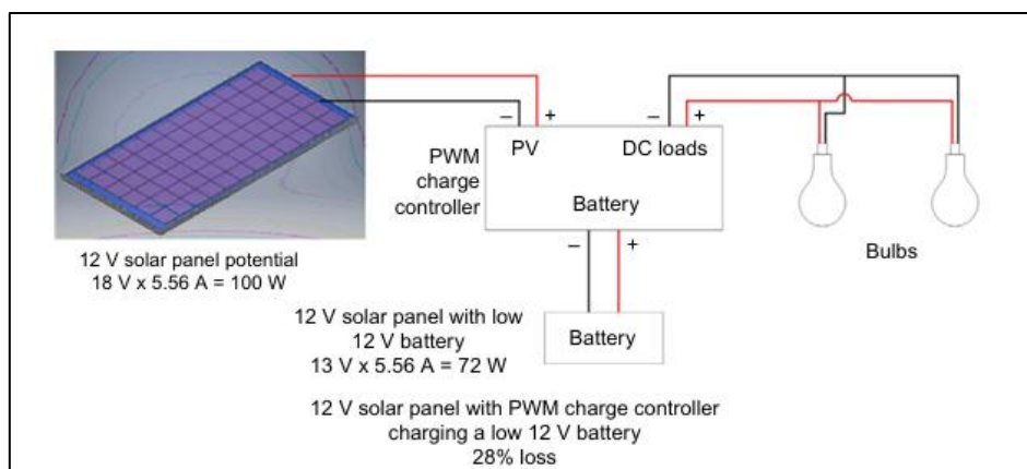
Figura 3.7 Pérdida de energía en una conexión de un módulo de 12V con una batería de 12V con un regulador de carga PWM
