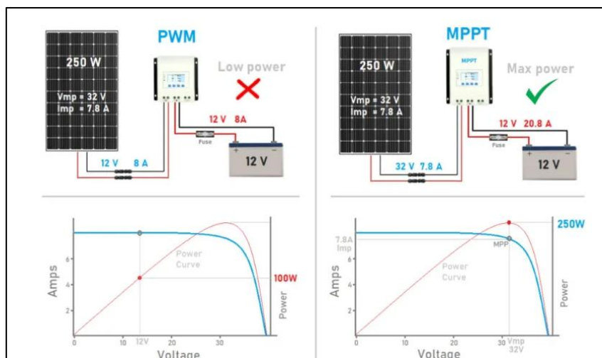
Figura 3.9 Comparación entre regulador PWM vs MPPT
