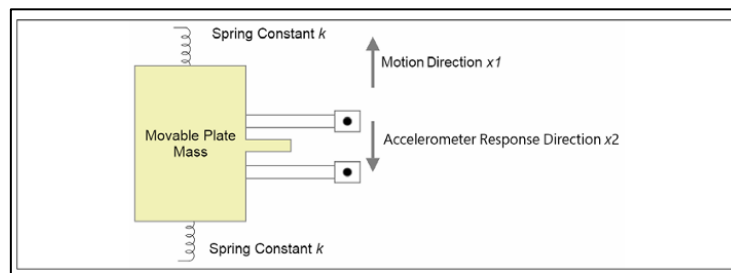
Figura 4.9 Principio de funcionamiento de un acelerómetro usando una masa suspendida por resortes
