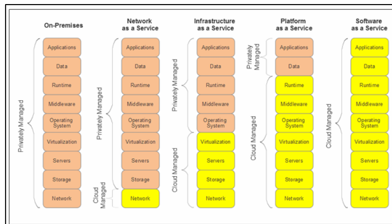
Figura 4.1 Modelos de arquitectura en la nube.
