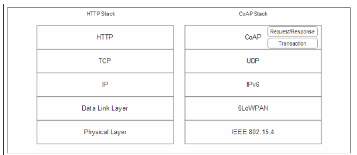
Figura 4.16 Comparación de estructura entre HTTP y CoAp
