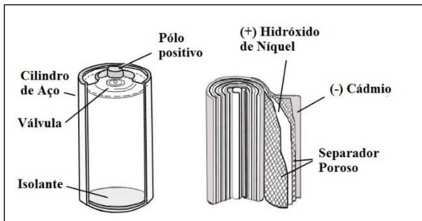
Figura 3.17 Batería cilíndrica de NiCd
