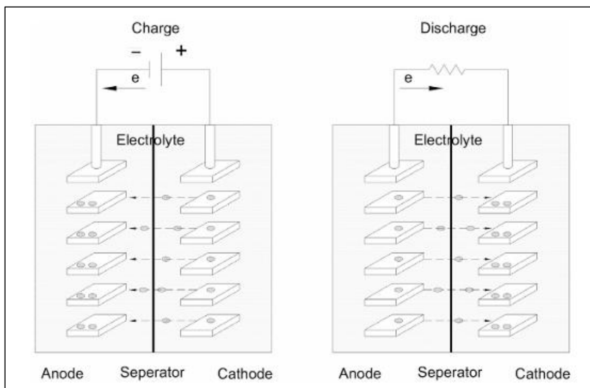
Figura 3.19 Principio de Operacion de la bateria de Ion-Litio
