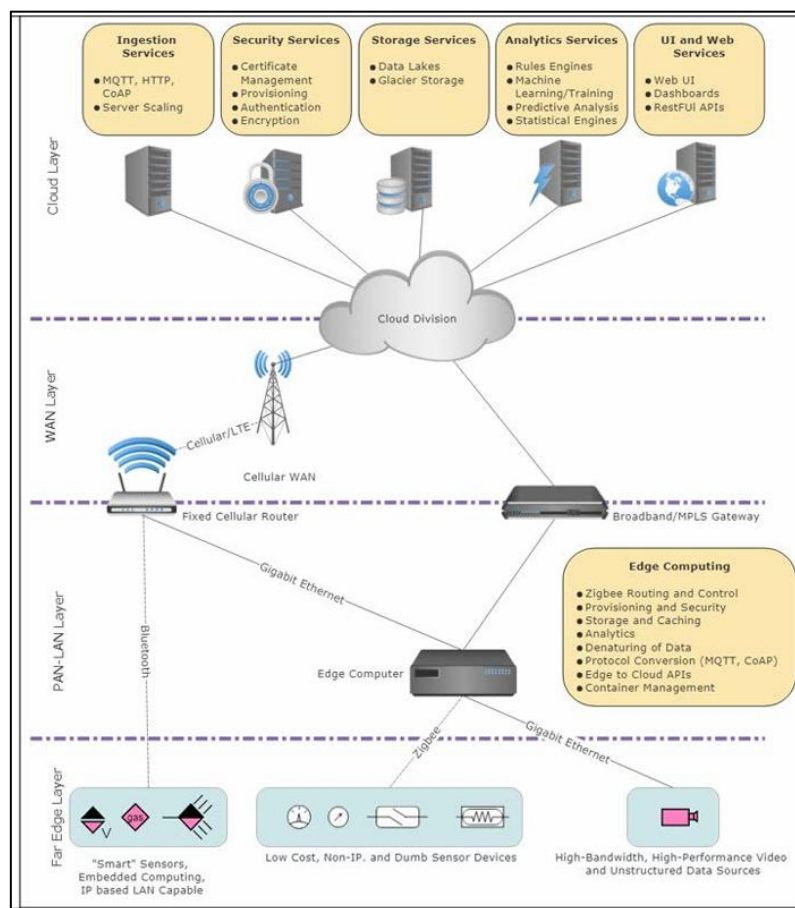
Figura 4.3 Ejemplo de arquitectura por capas de un sistema de computación IoT-Edge.
