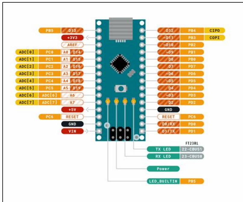
Figura 4.5 Esquemático y distribución de pines del Arduino Nano
