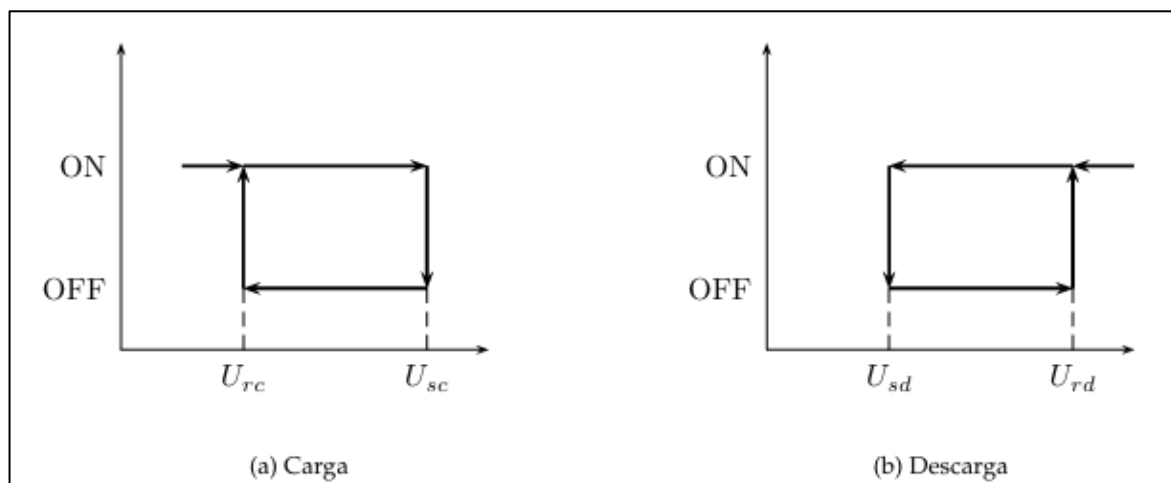
Figura 3.6 Histéresis de protección frente a sobrecarga y sobredescarga en un regulador
