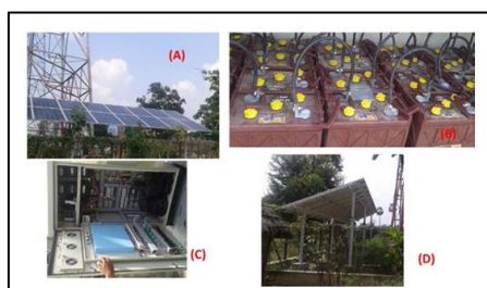
Figura 3.24 Sistema fotovoltaico de apoyo para torres de telecomunicaciones: (A) campo solar, (B) banco de baterías, (C) regulador de carga y (D) sistema de montaje de los módulos solares.
