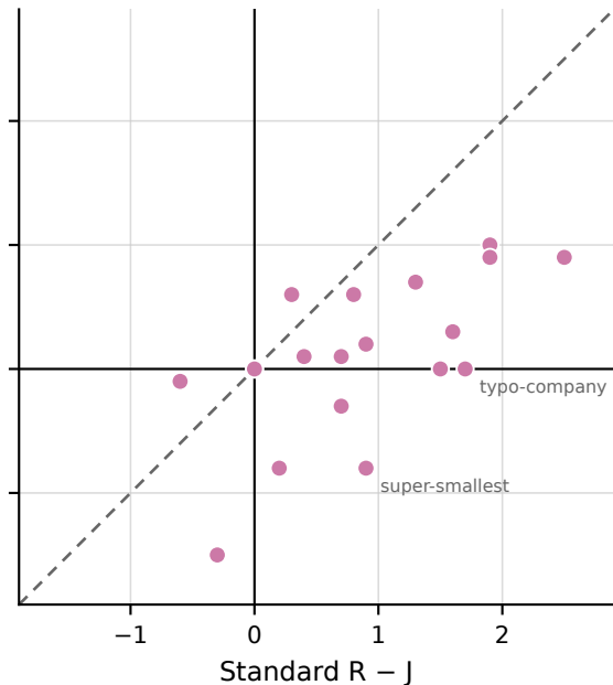
Gemma-3-27B-it
