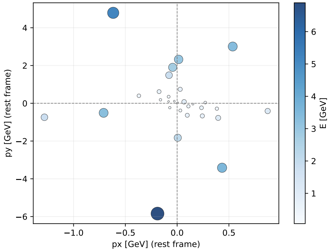
Quark jet mult=31
