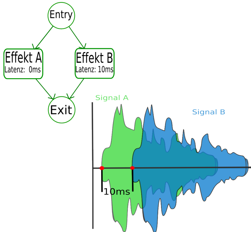
Abbildung 6: Darstellung des Latenzproblem: die Signalausgabe aus "Effekt B" ist um 10 ms verzögert
