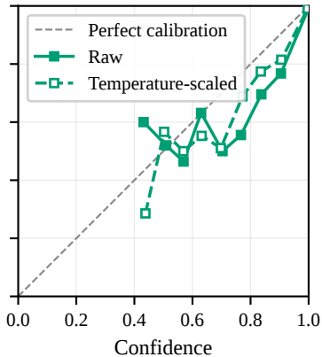
(b) EfficientNet-B0
