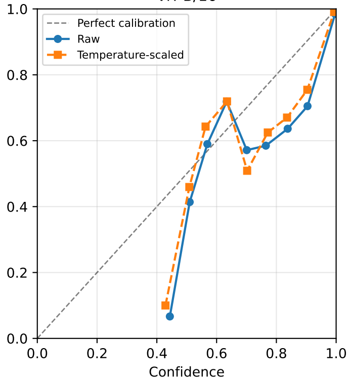
ViT-B/16
