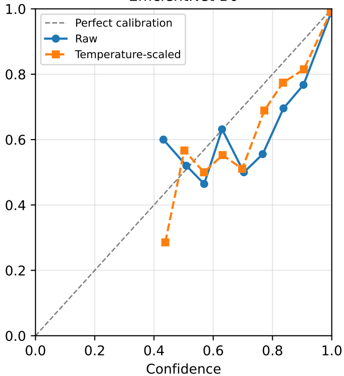
EfficientNet-B0
