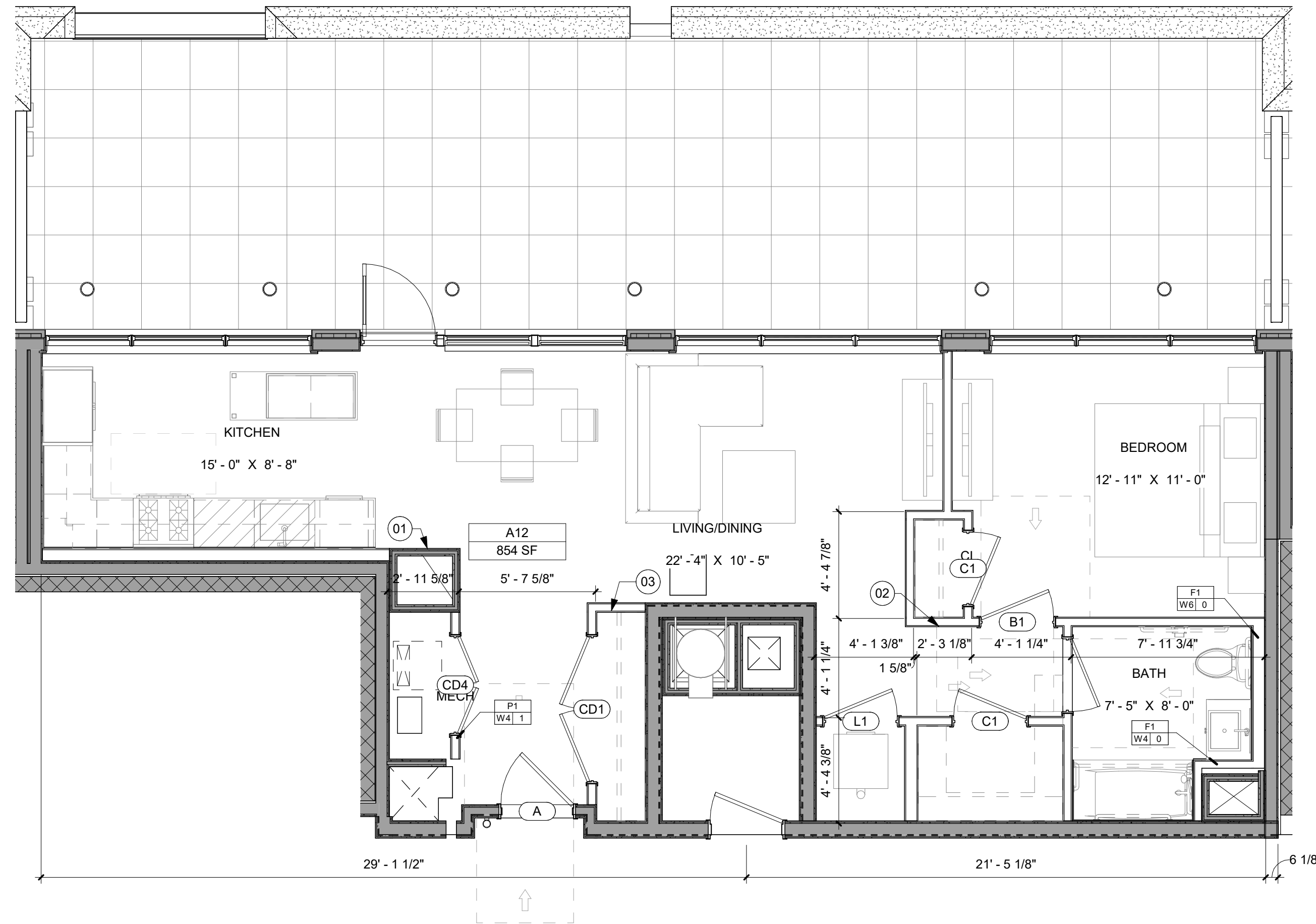
10 UNIT TYPE - A12 SCALE: 1/4" = 1'-0"
