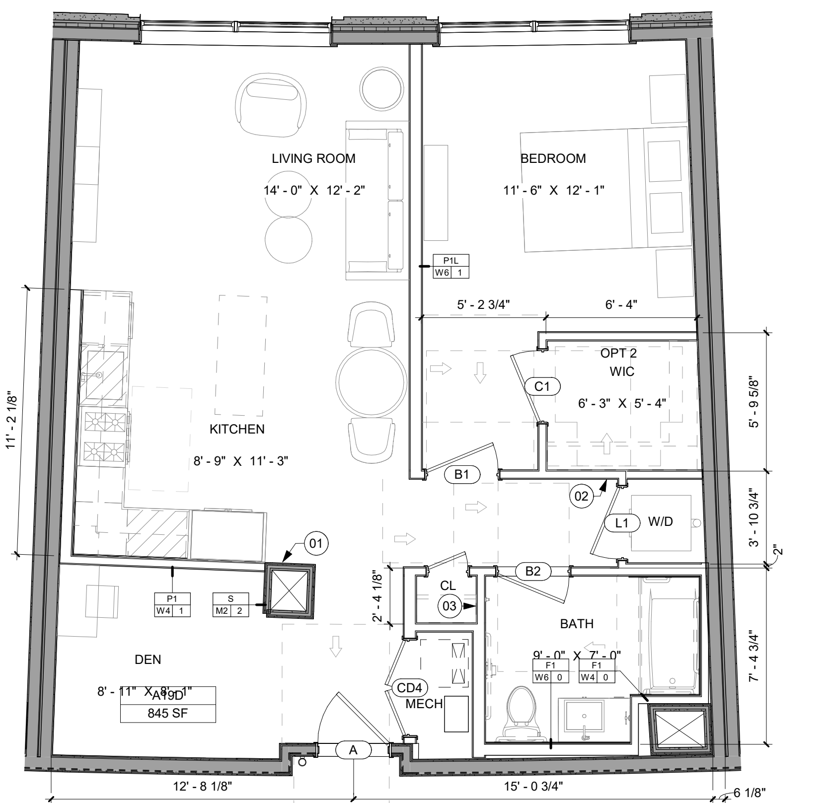
3 UNIT TYPE - A19D SCALE: 1/4" = 1'-0"
