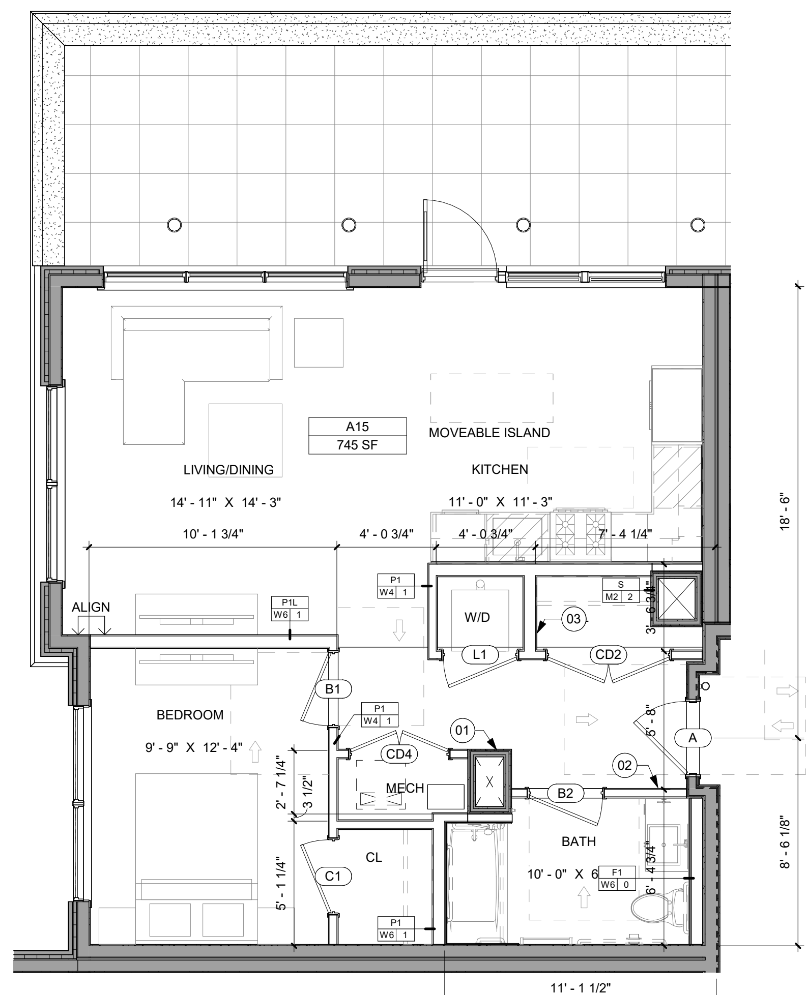
7 UNIT TYPE - A15 SCALE: 1/4" = 1'-0"
