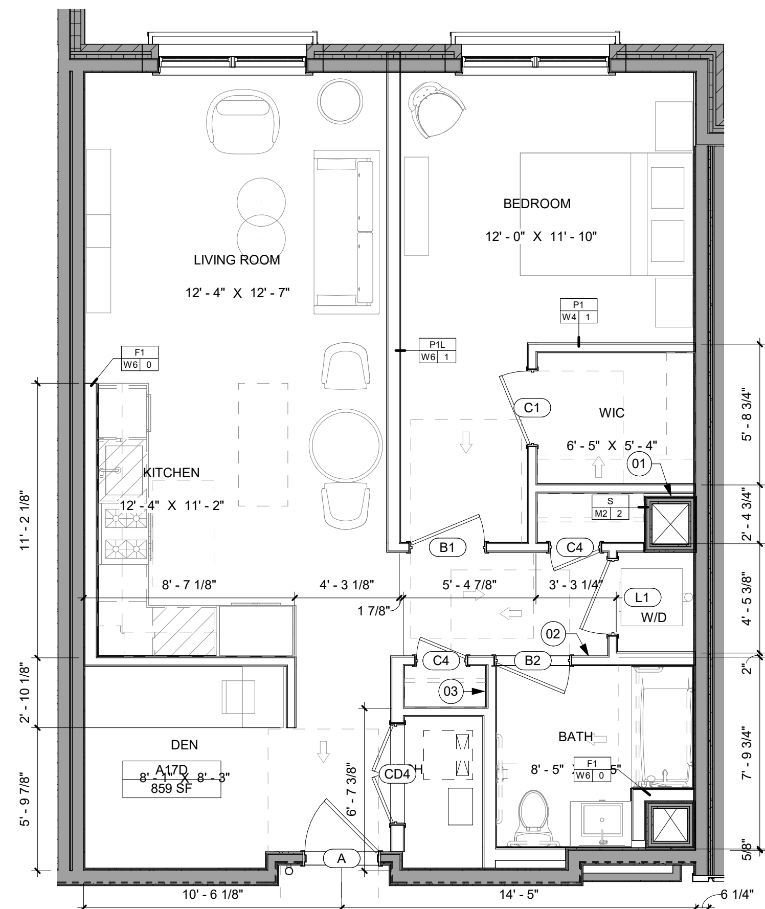
5 UNIT TYPE - A17D SCALE: 1/4" = 1'-0"
