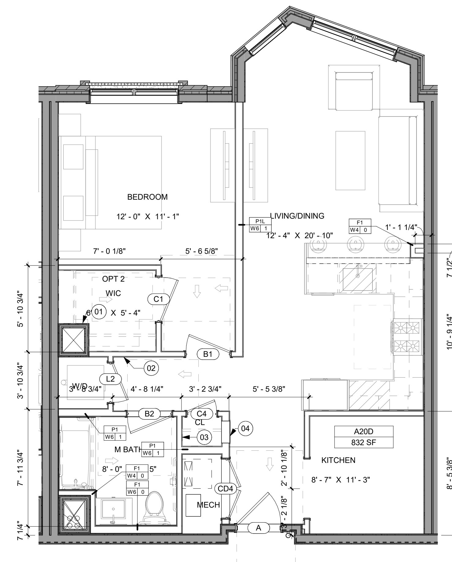
2 UNIT TYPE - A20D SCALE: 1/4" = 1'-0"
