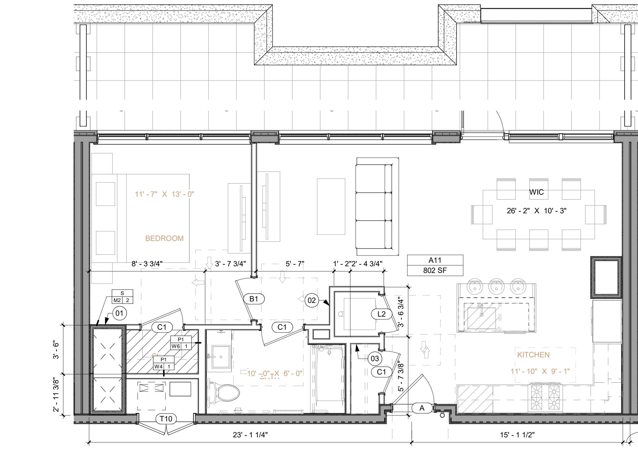
11 UNIT TYPE - A11 SCALE: 1/4" = 1'-0"
