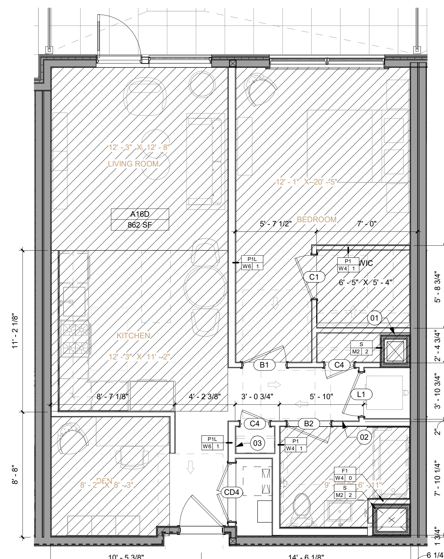
6 UNIT TYPE - A16D SCALE: 1/4" = 1'-0"
