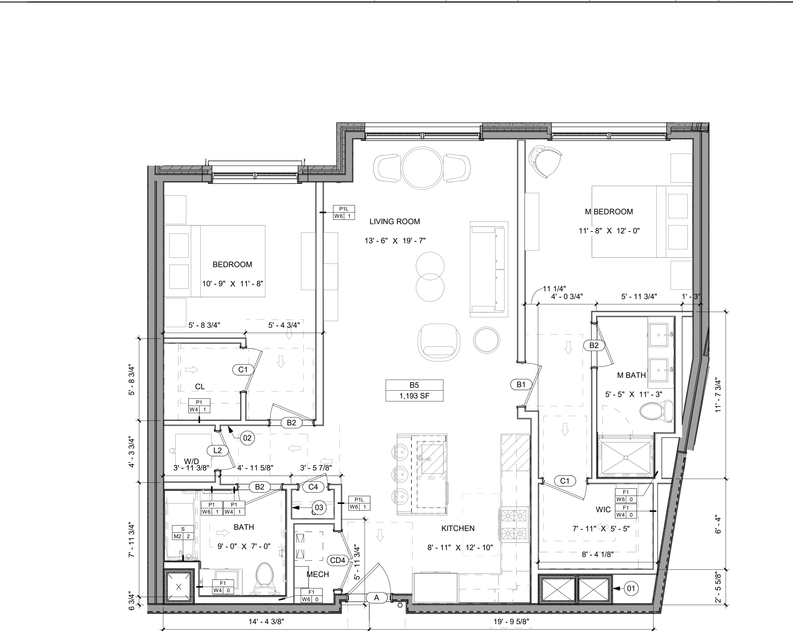
3 UNIT TYPE - B5 SCALE: 1/4" = 1'-0"
