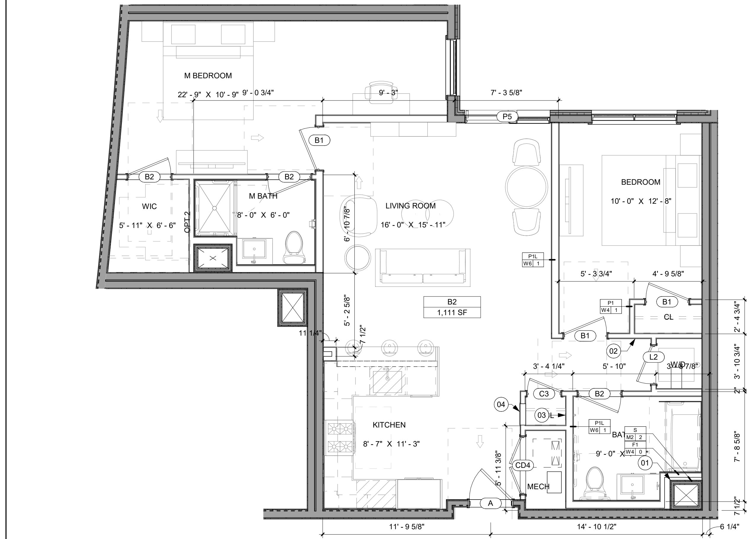
7 UNIT TYPE - B2 SCALE: 1/4" = 1'-0"
