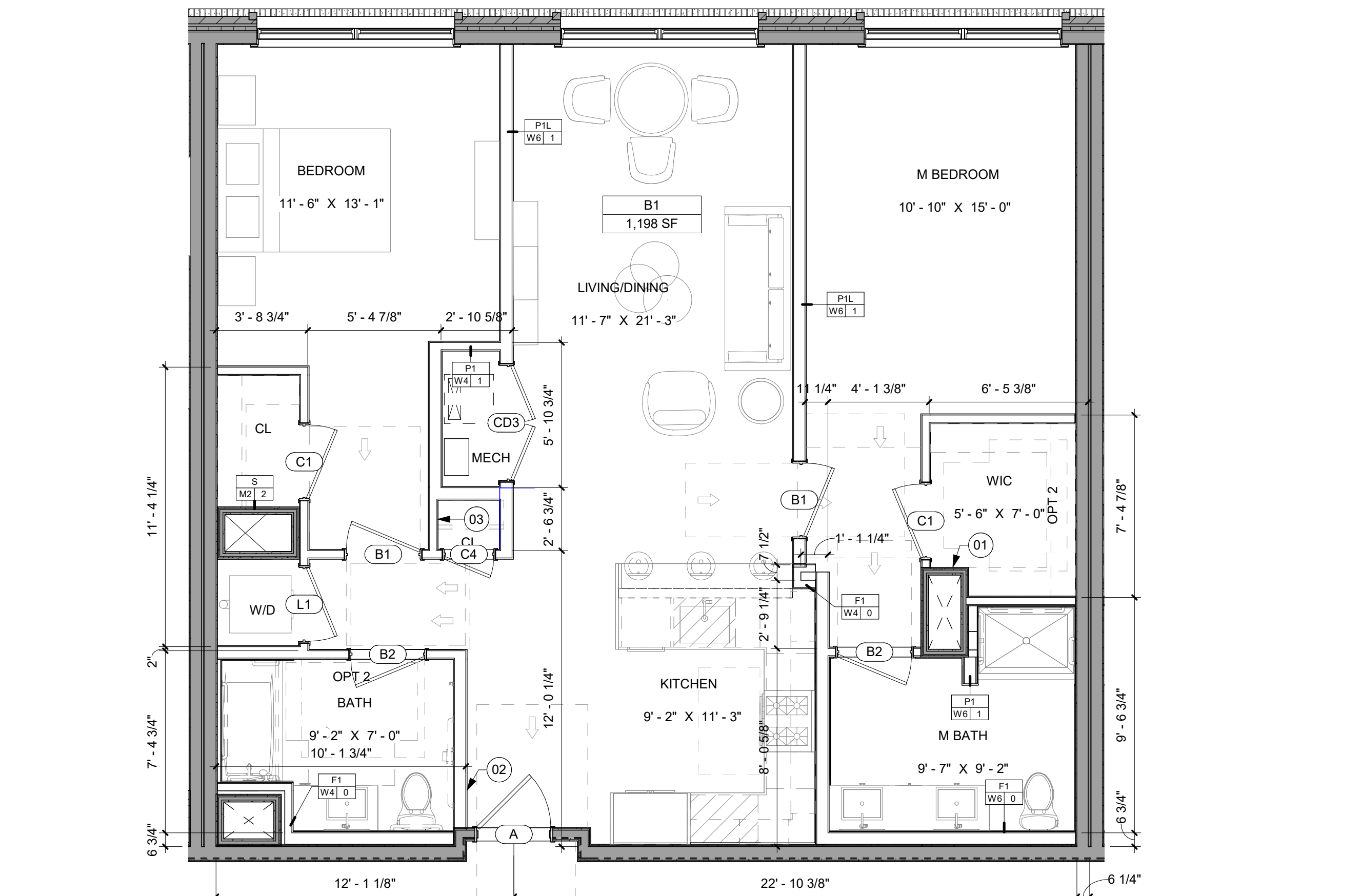
37 UNIT TYPE - B1 SCALE: 1/4" = 1'-0"
