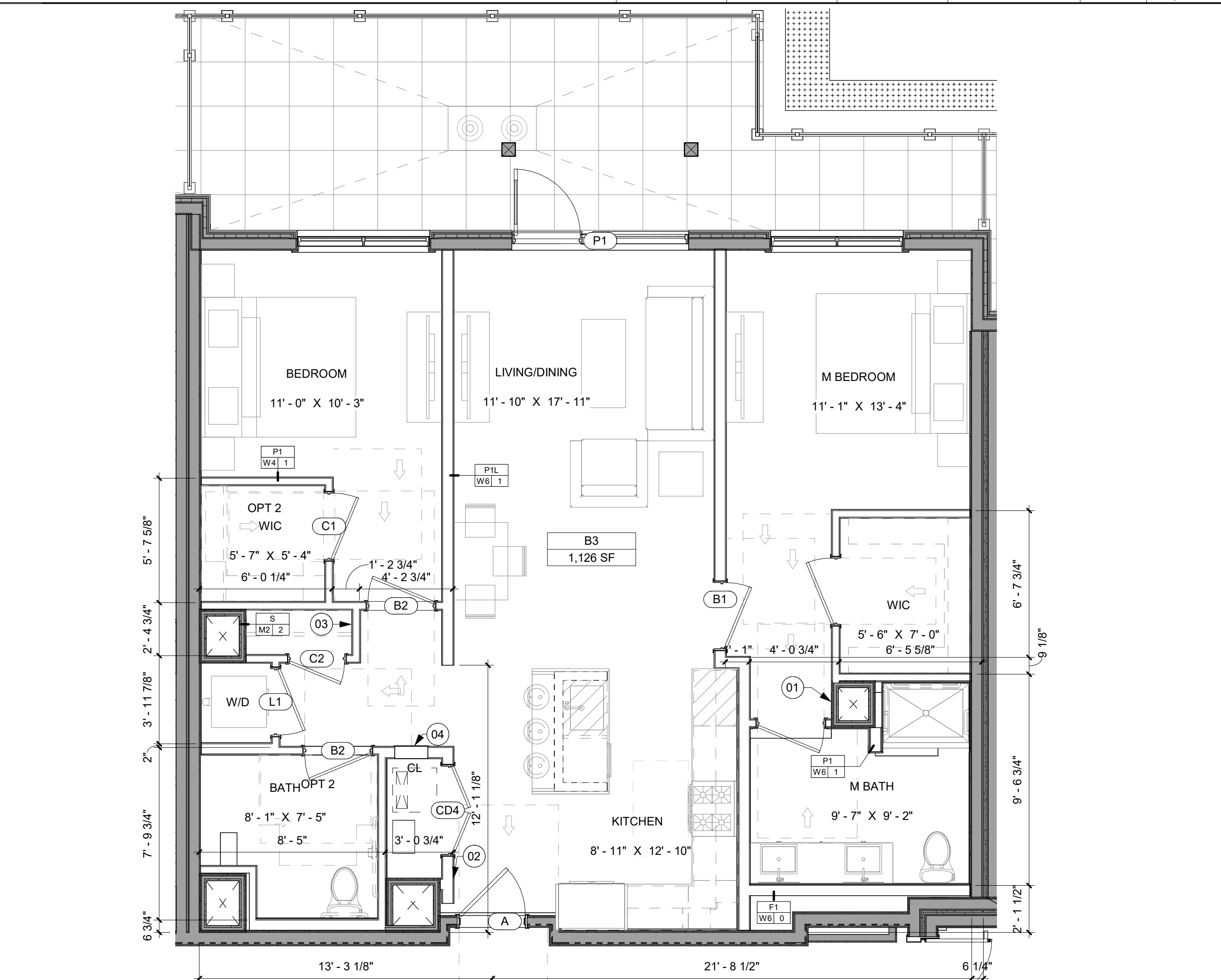
6 UNIT TYPE - B3 SCALE: 1/4" = 1'-0"
