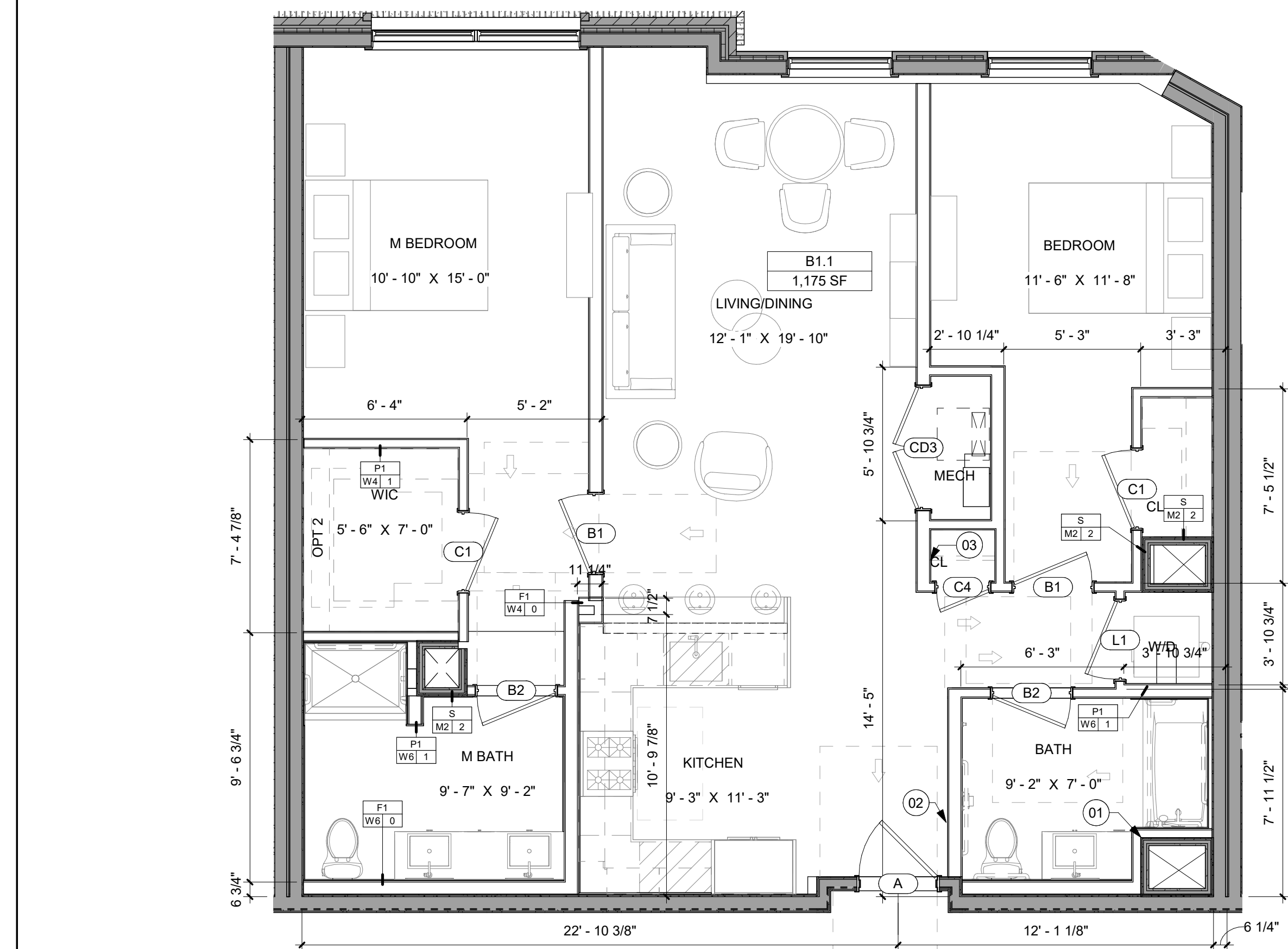
8 UNIT TYPE - B1.1 SCALE: 1/4" = 1'-0"
