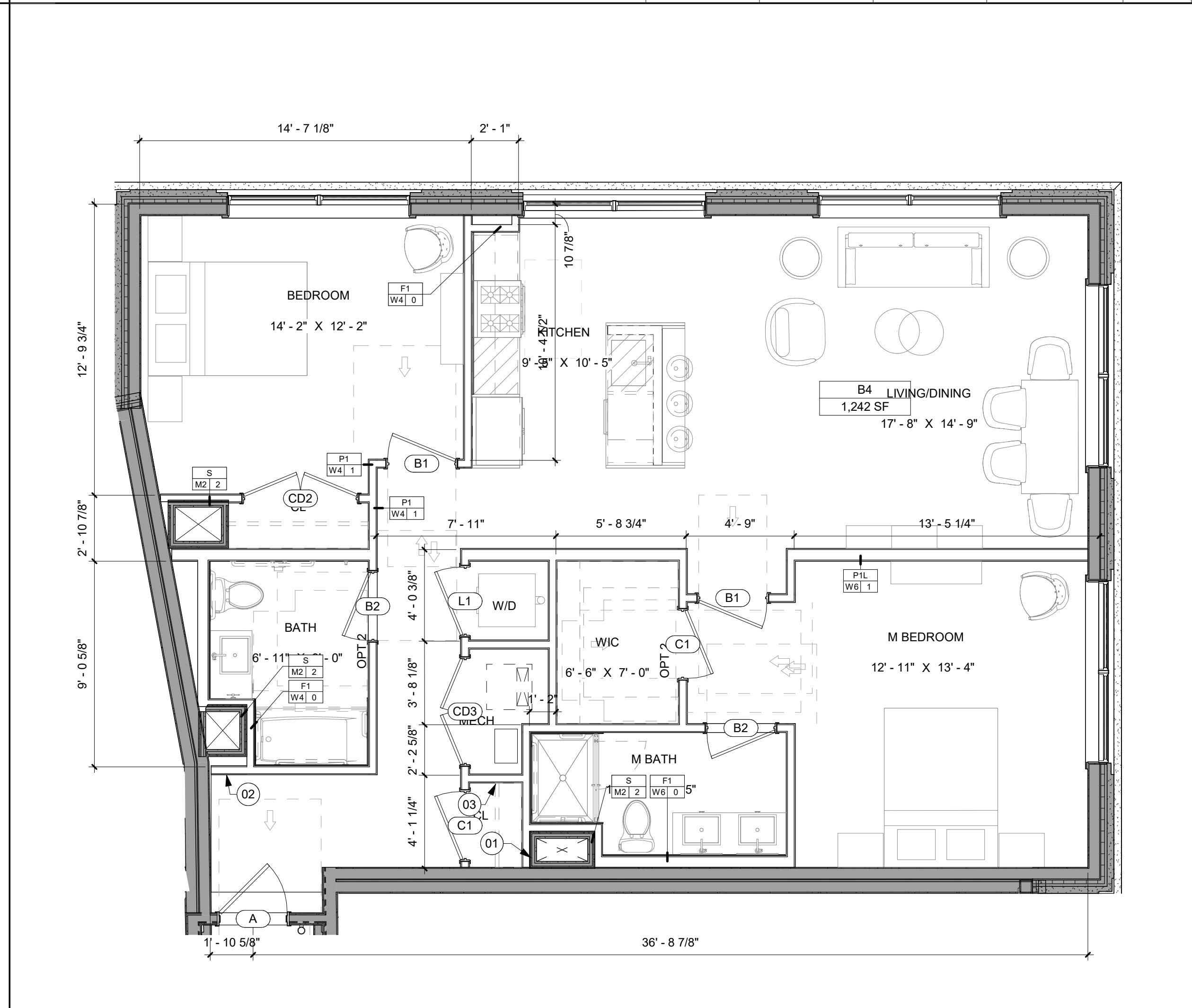
4 UNIT TYPE - B4 SCALE: 1/4" = 1'-0"
