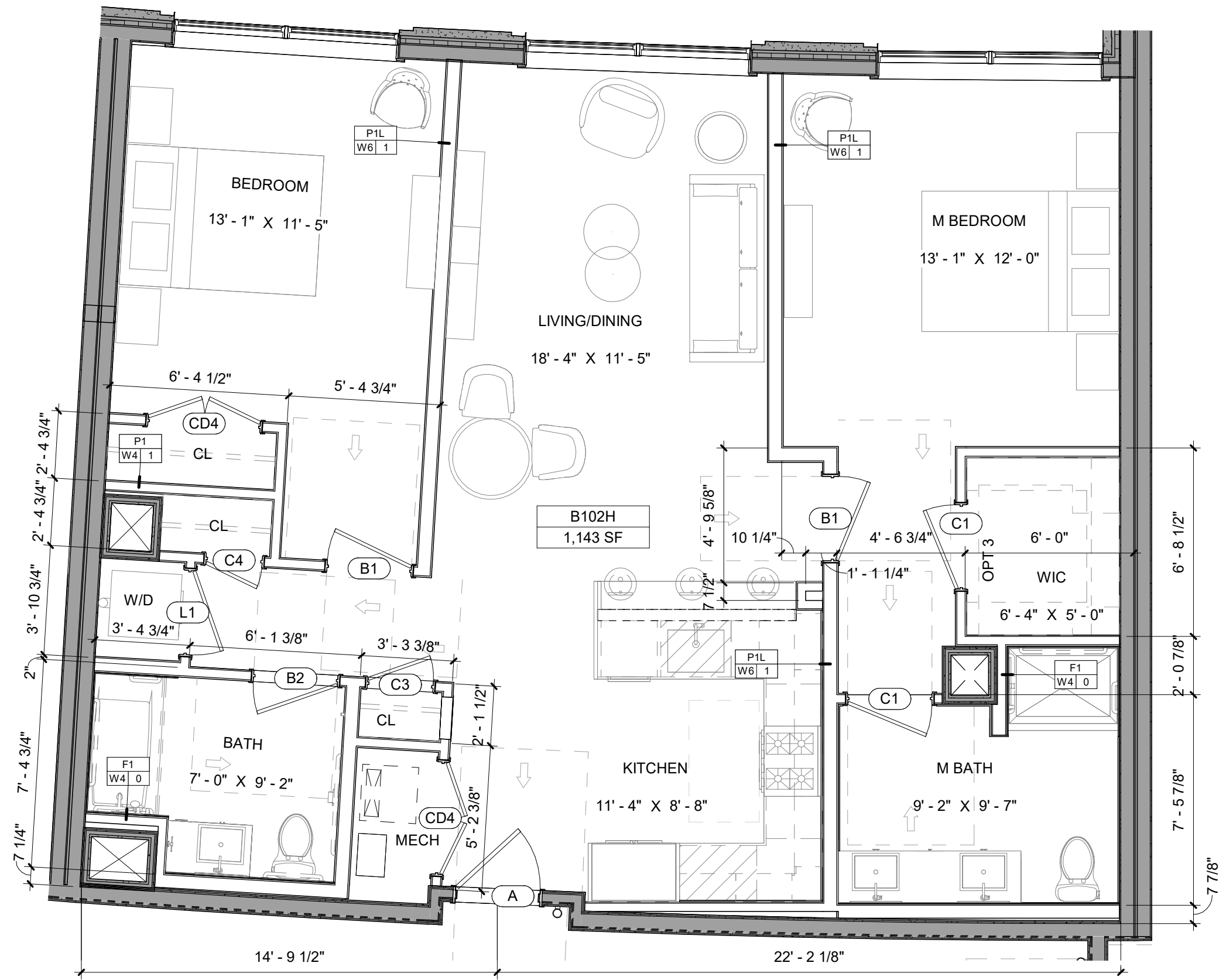
4 UNIT TYPE - B102H SCALE: 1/4" = 1'-0"
