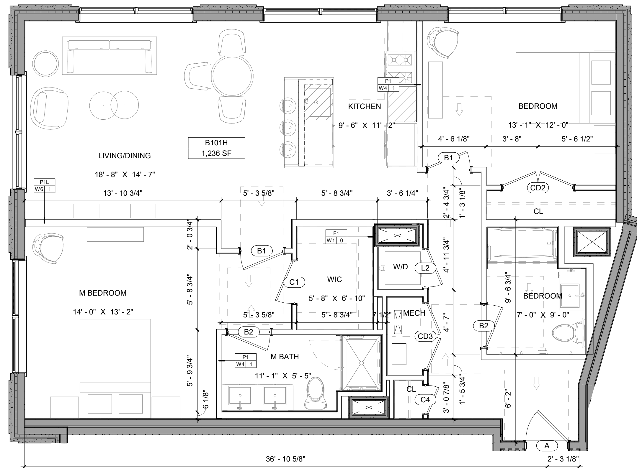
5 UNIT TYPE - B101H SCALE: 1/4" = 1'-0"
