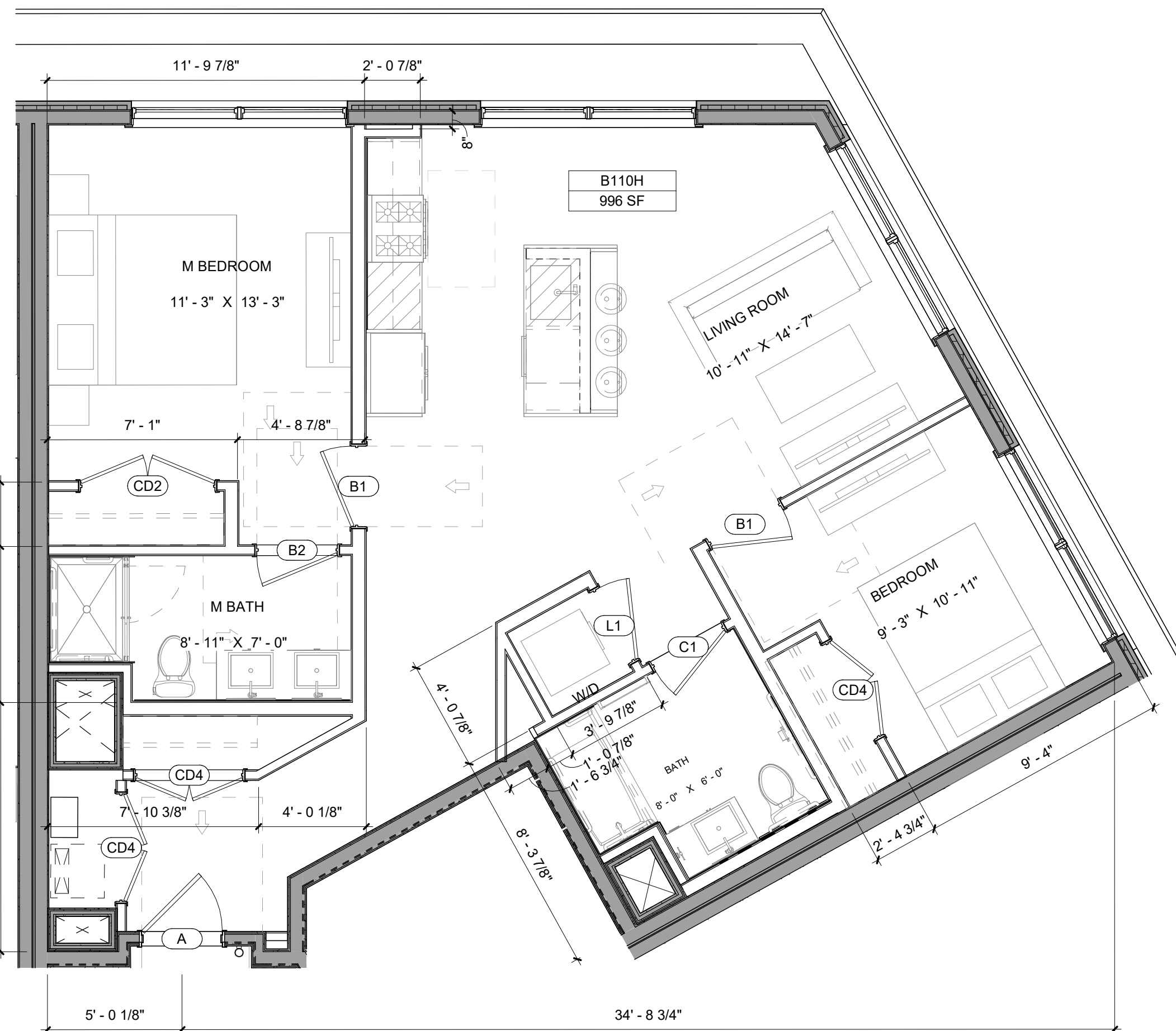
3 UNIT TYPE - B110H SCALE: 1/4" = 1'-0"
