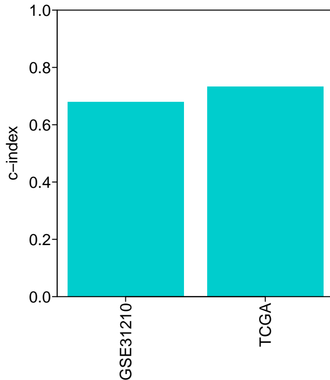
c-index
